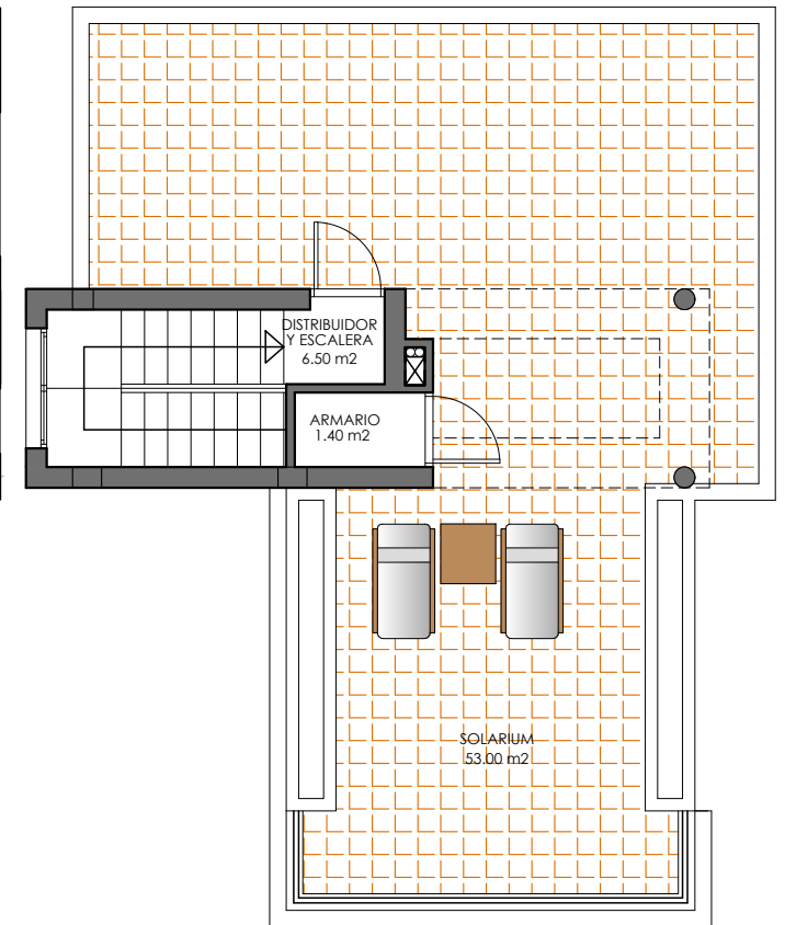
CUBIERTA
