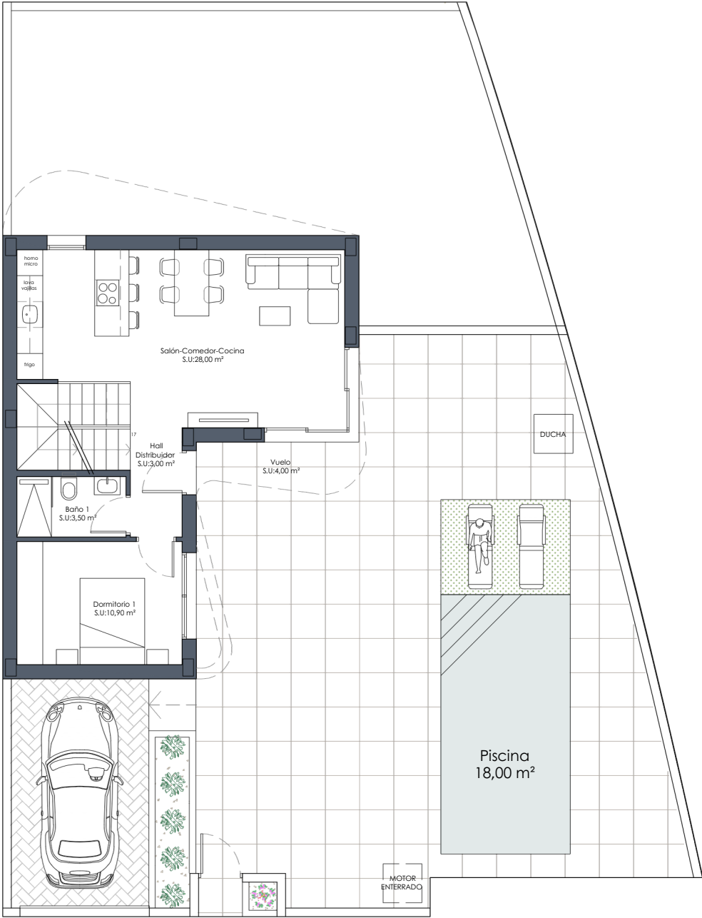
PLANTA BAJA
