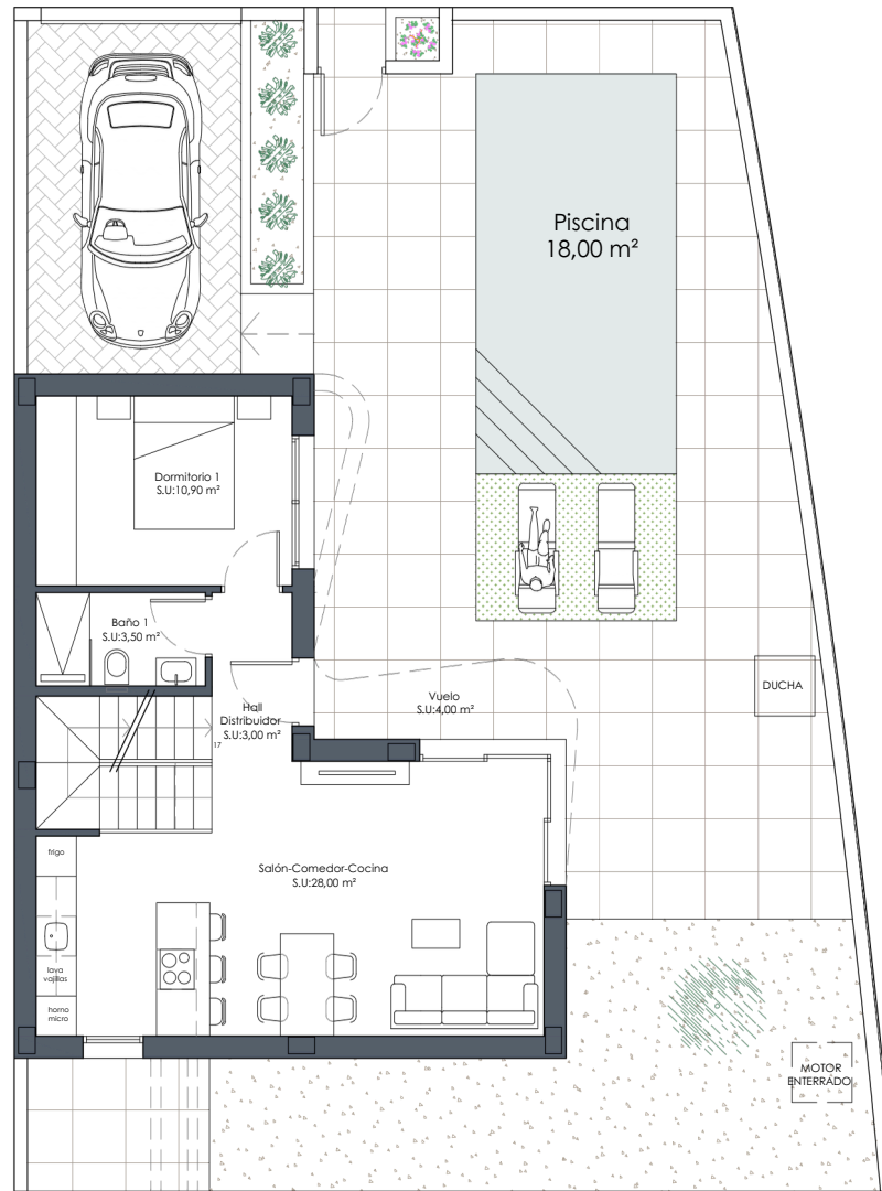
PLANTA BAJA
