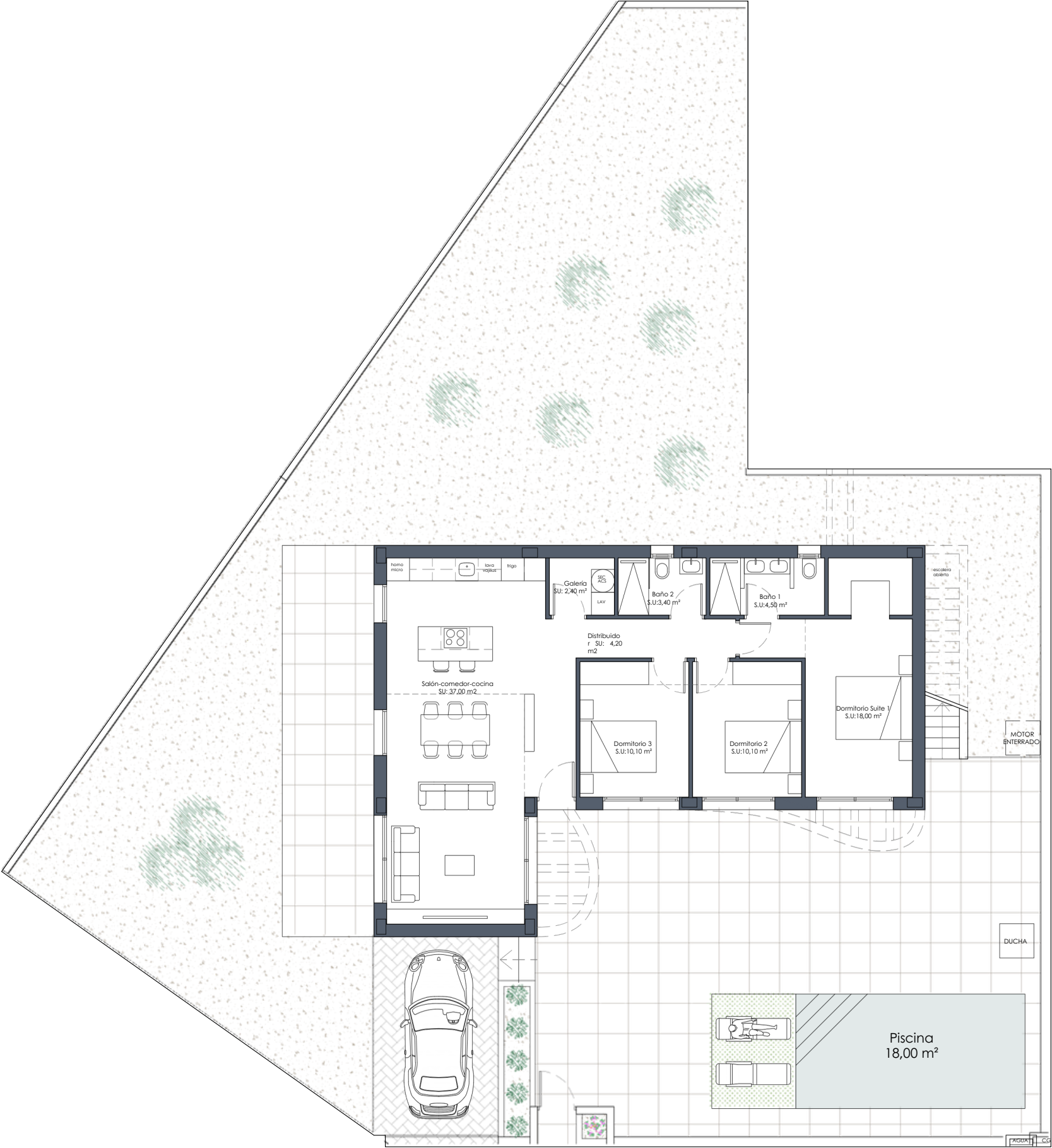
PLANTA BAJA
