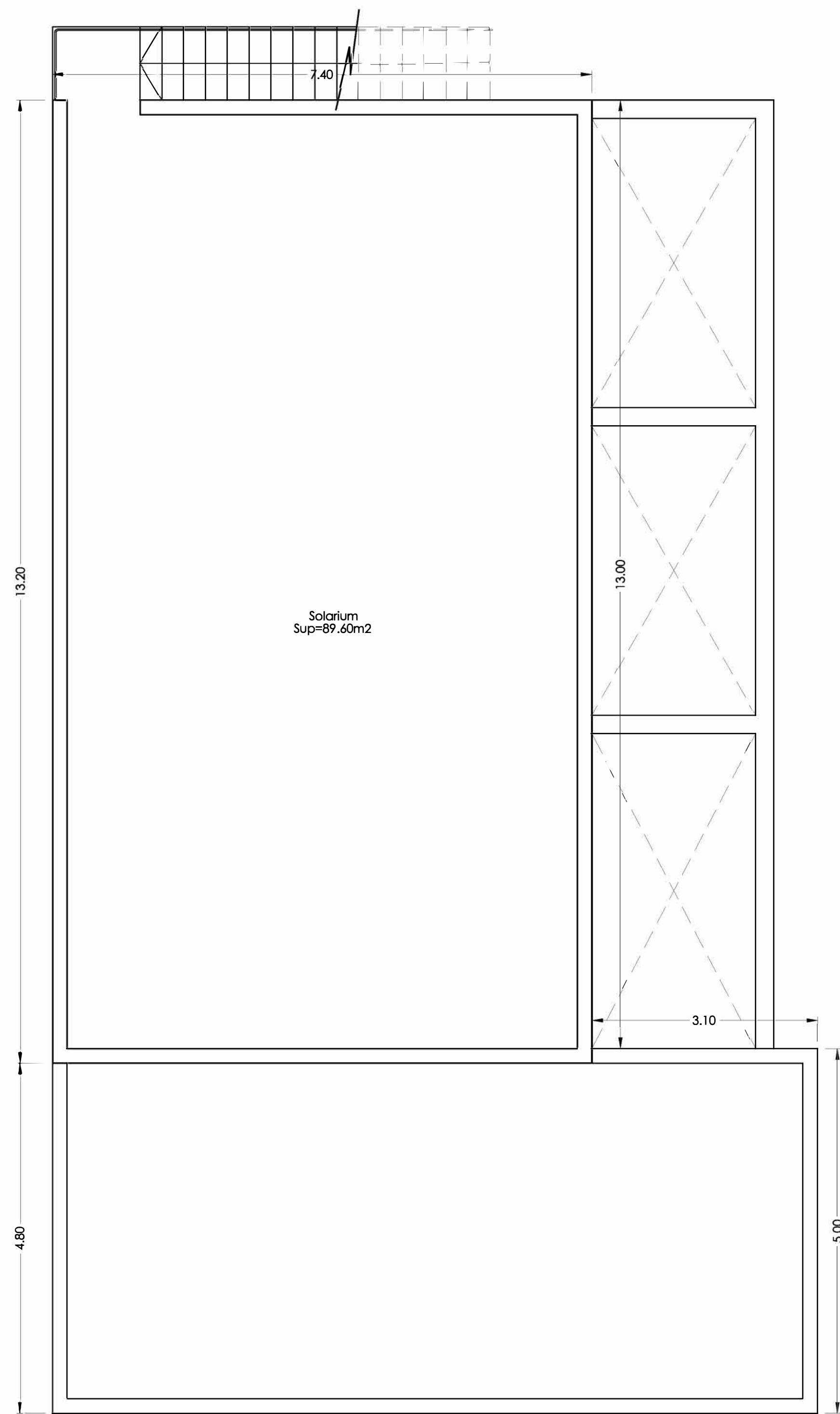
PLANTA SOLARIUM
