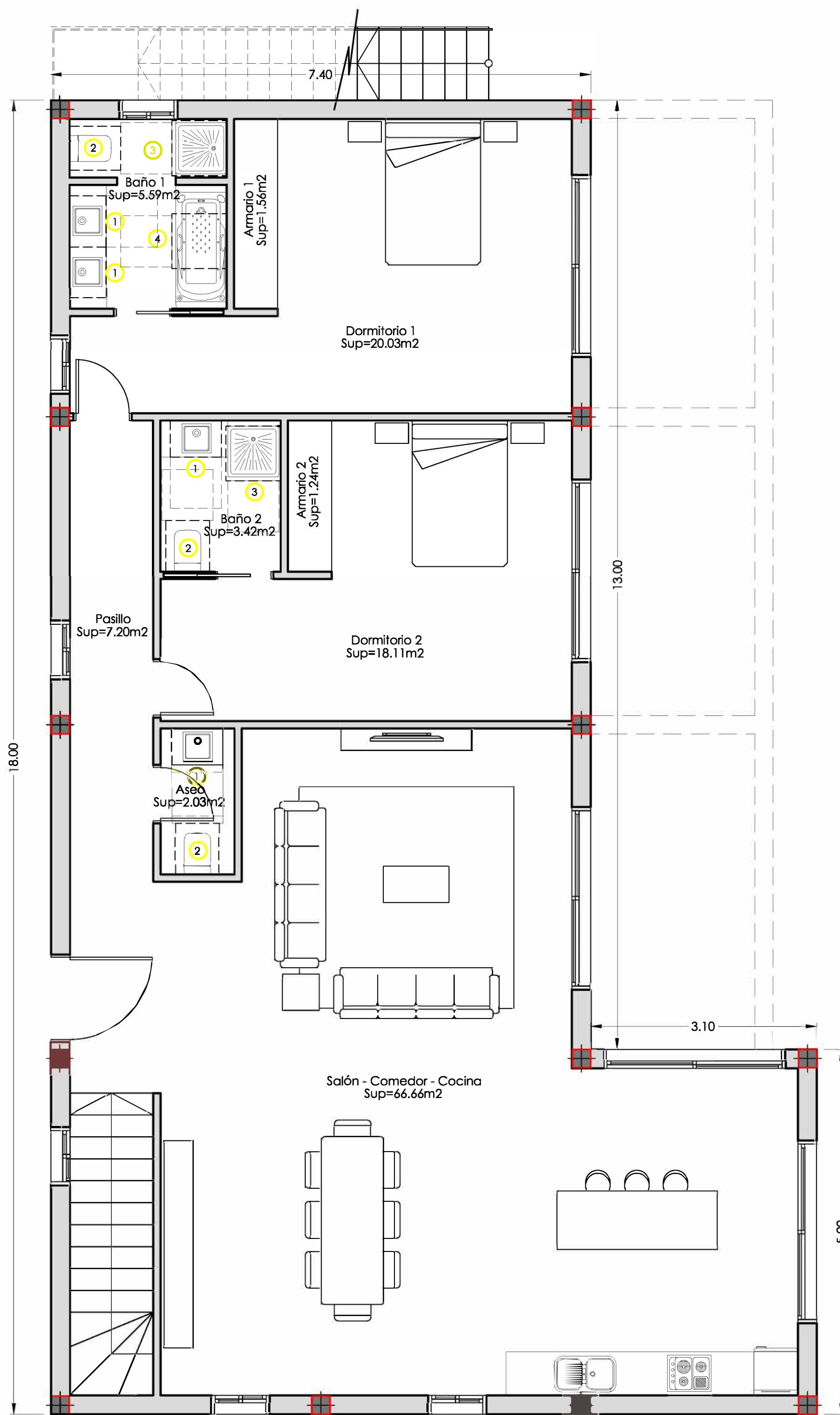
PLANTA BAJA
