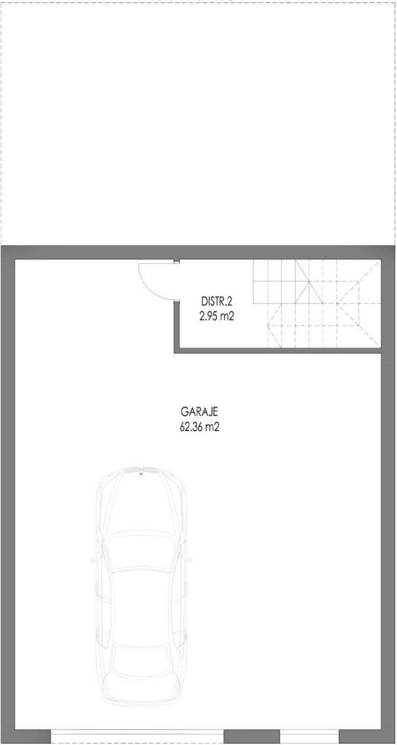
PLANTA PRIMERA
