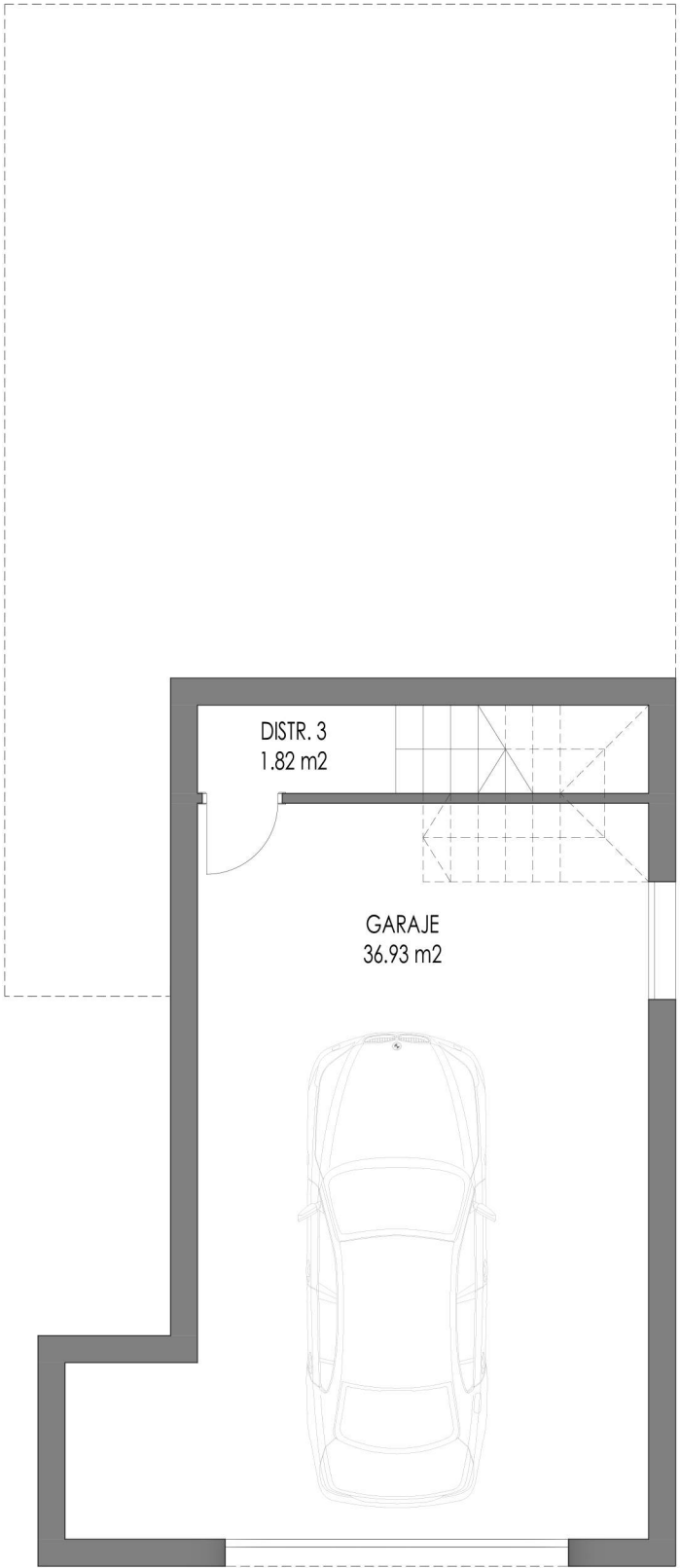
PLANTA SÓTANO
