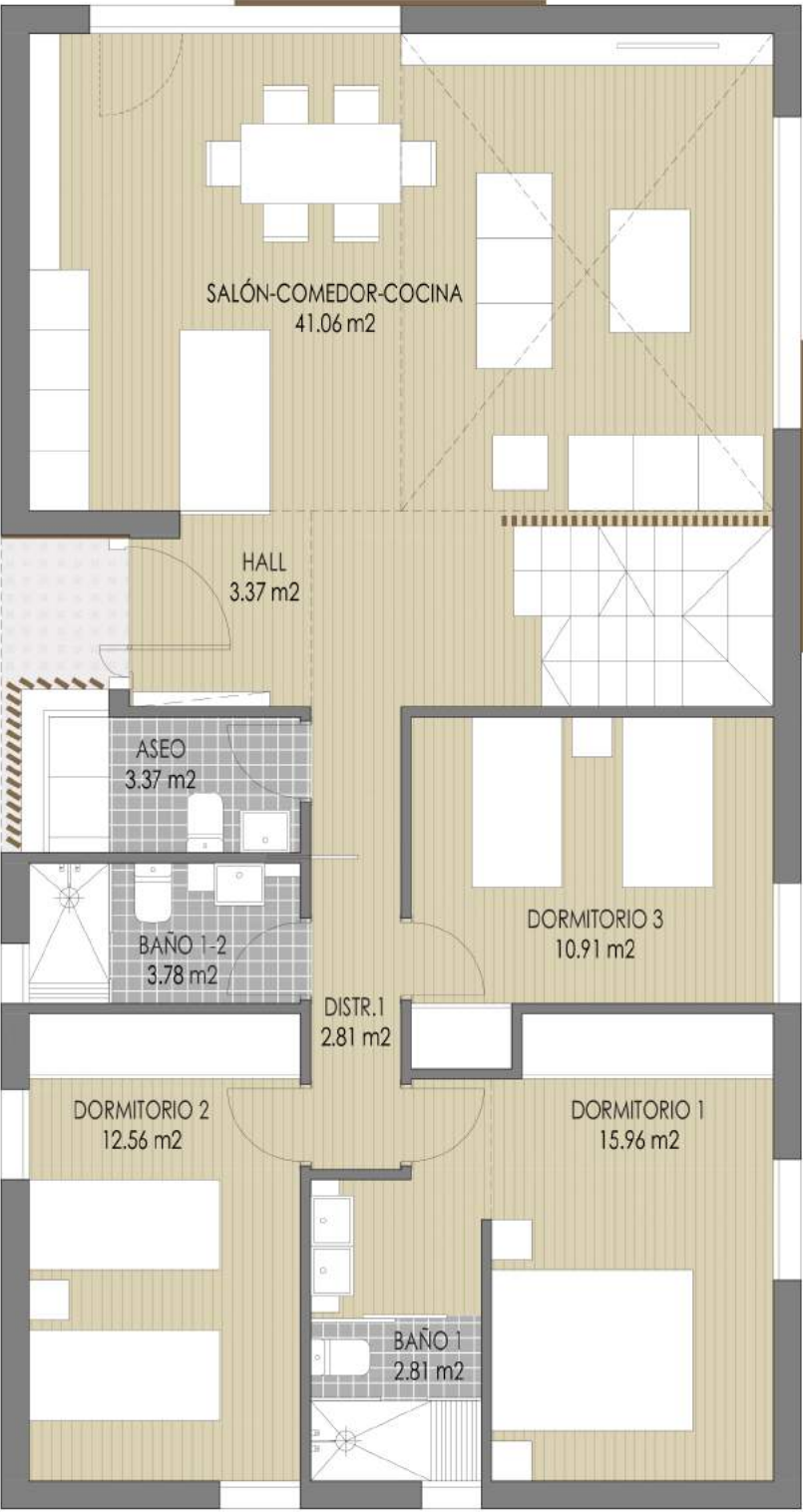
PLANTA BAJA
