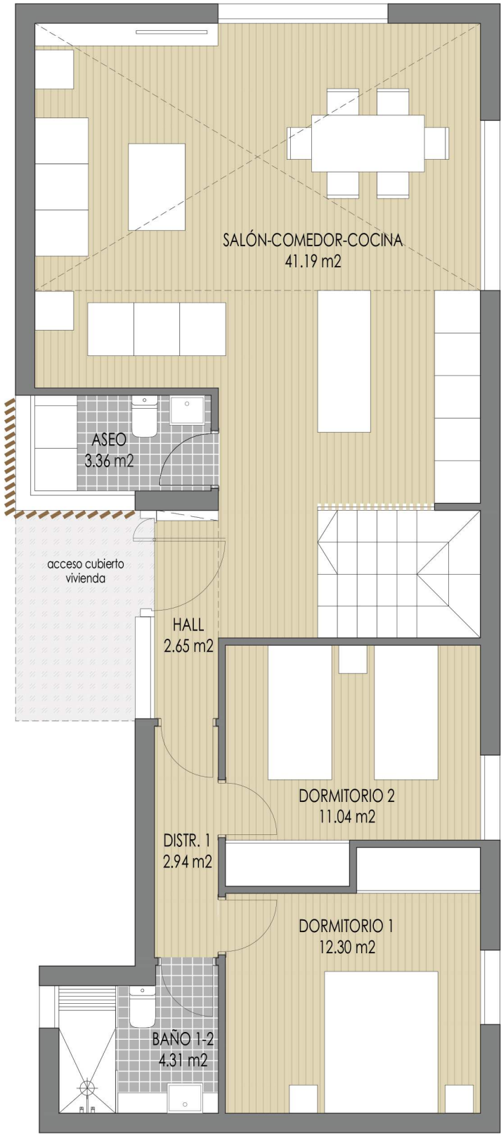
PLANTA BAJA
