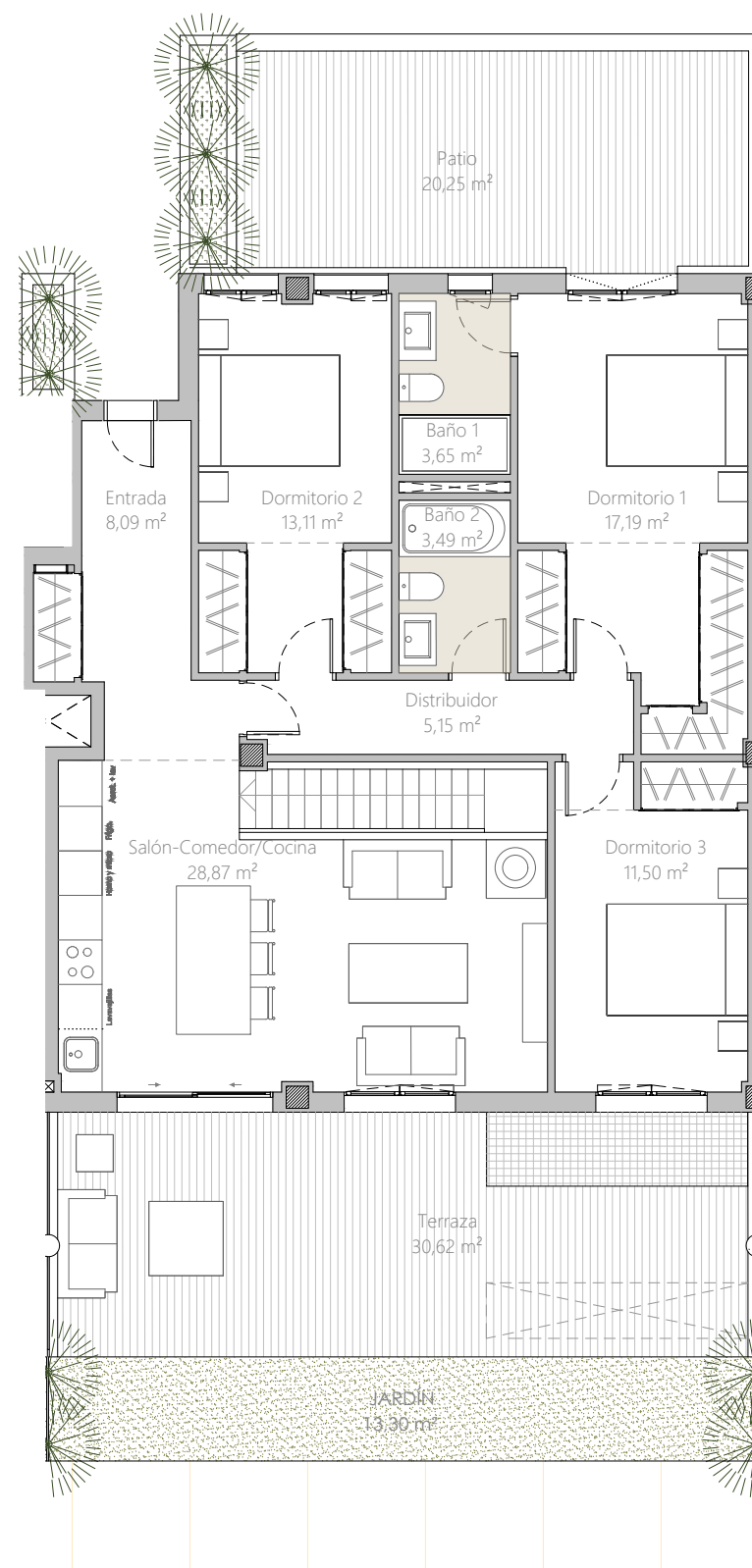
PLANTA BAJA
