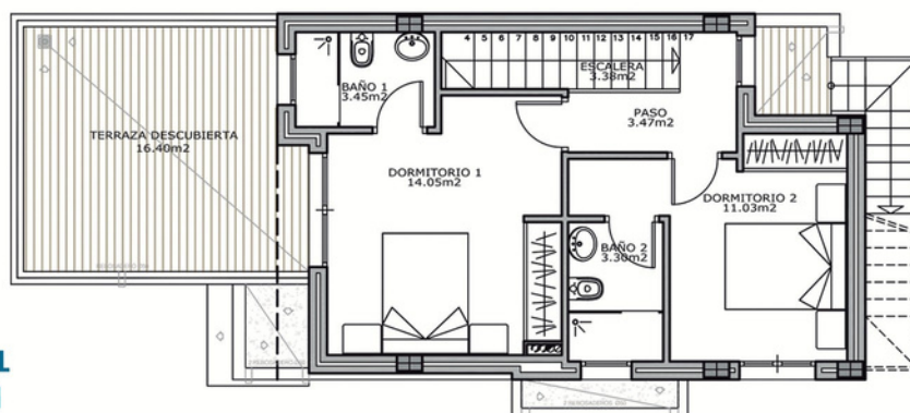
PLANTA PRIMERA
