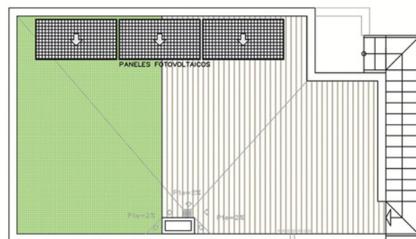
PLANTA CUBIERTAS
