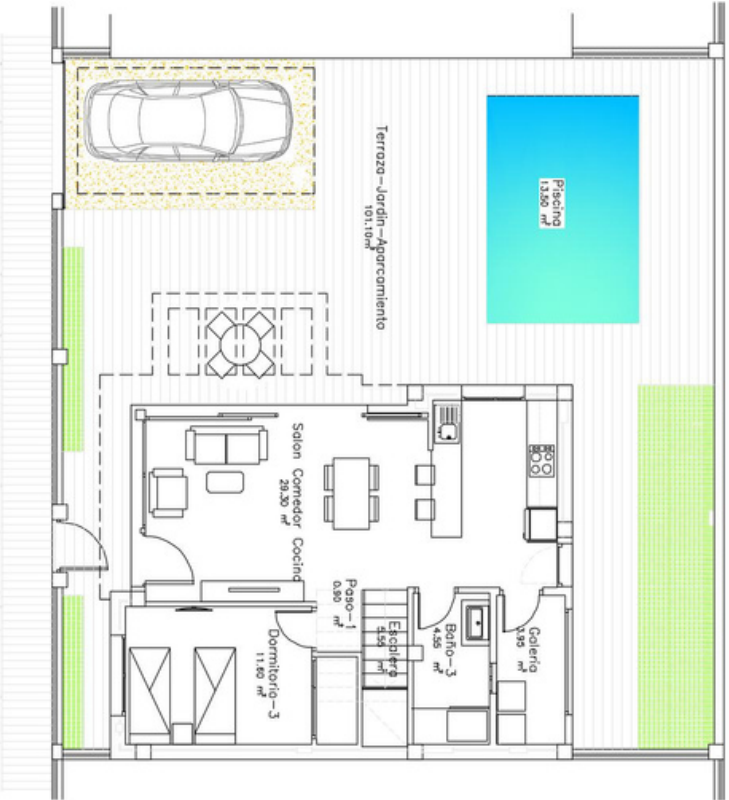
PLANTA BAJA.
