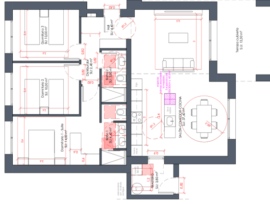
PLANTA BAJA
