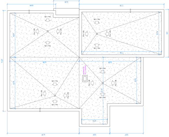
PLANTA CUBIERTA
