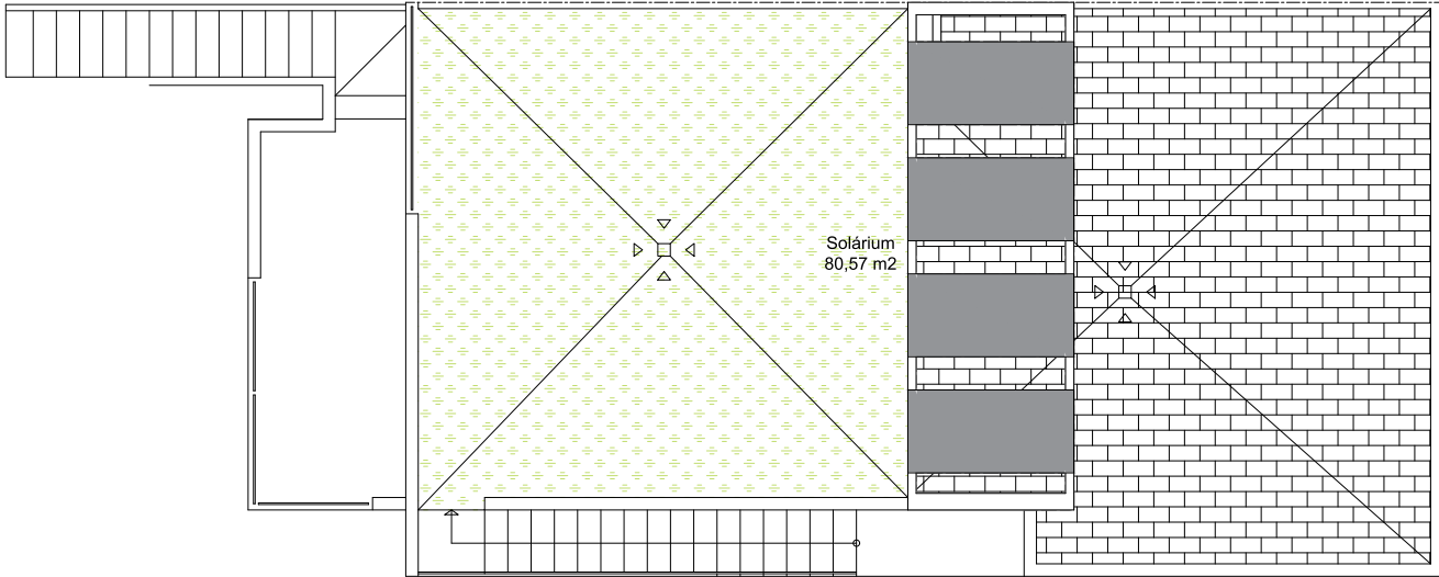
PLANTA SOLARIUM
