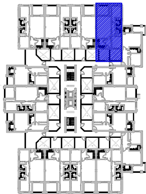
PLANTA SEGUNDA
