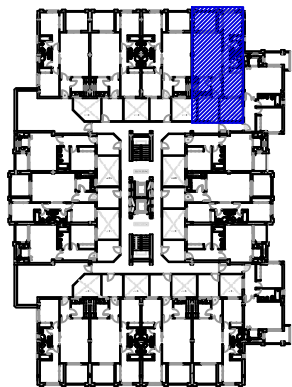
PLANTA PRIMERA
