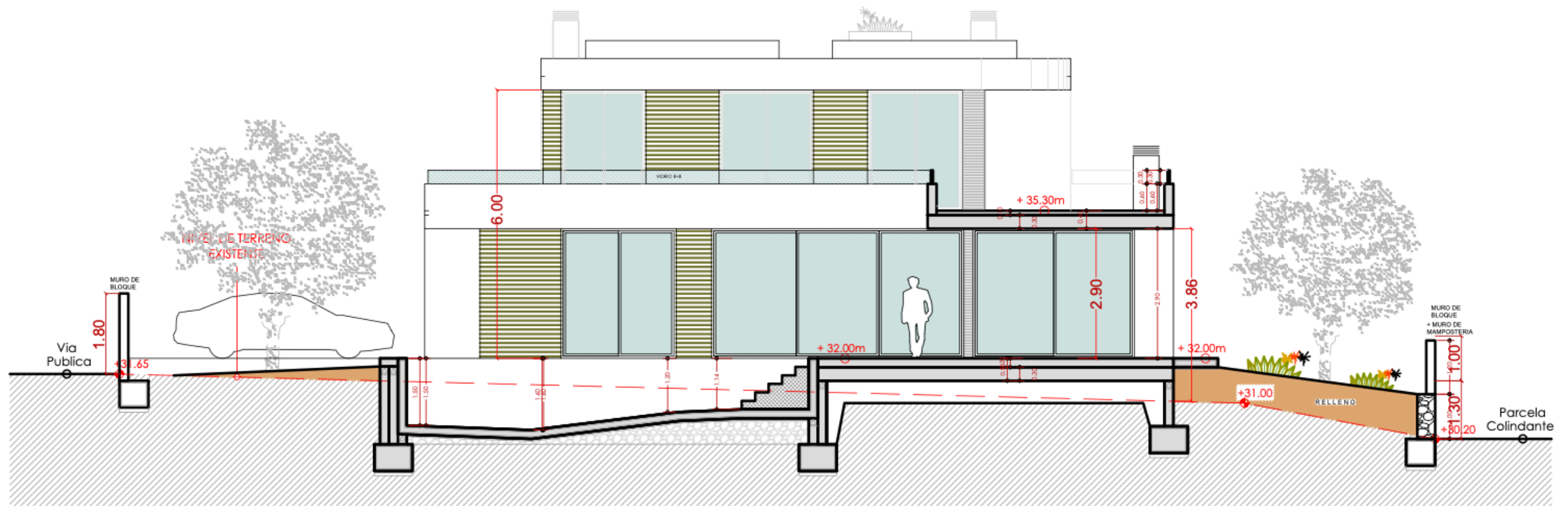
SECCIÓN A-A'
