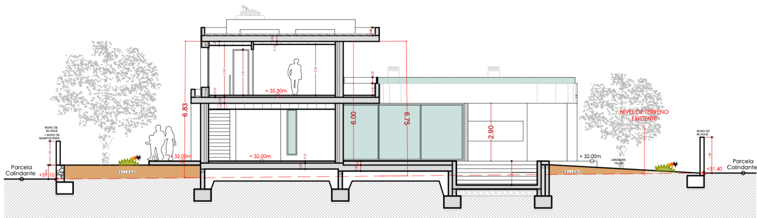
SECCIÓN C-C'
