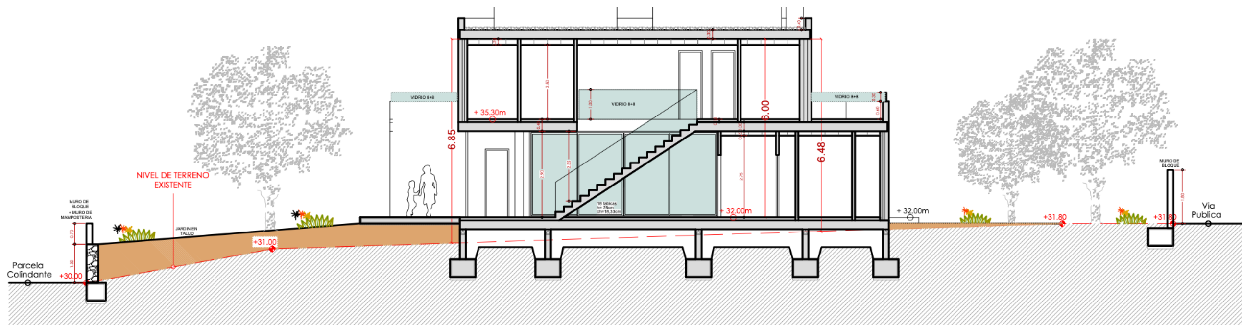
SECCIÓN B-B'
