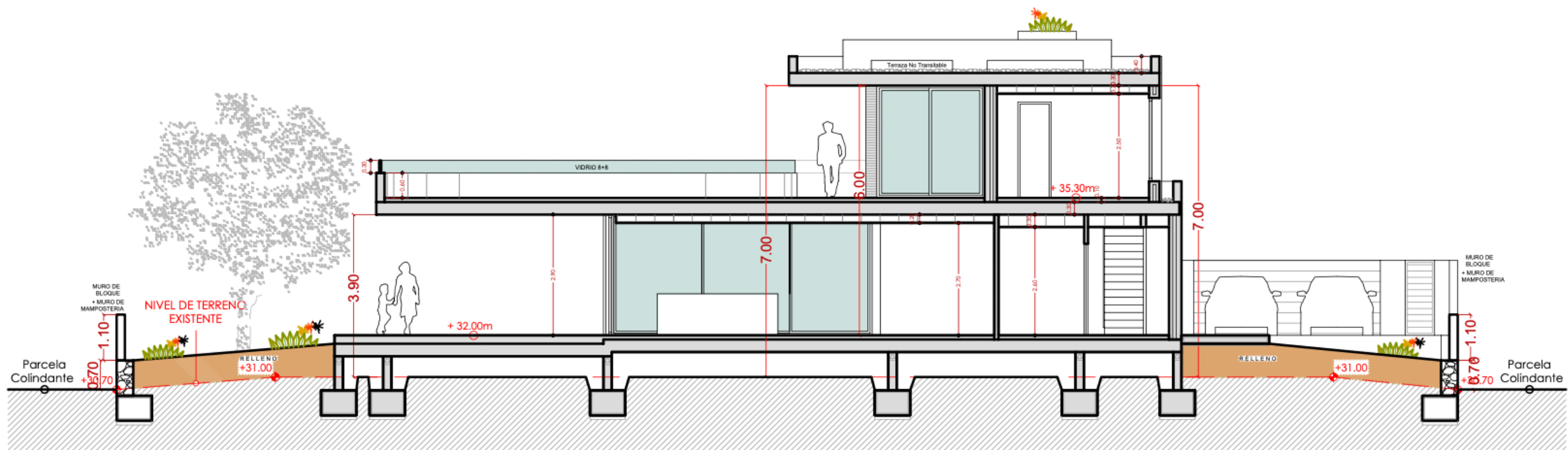
SECCION D'-D
