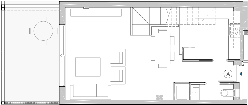
Planta primera
