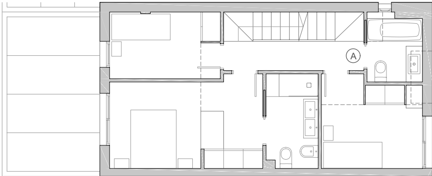
Planta segunda
