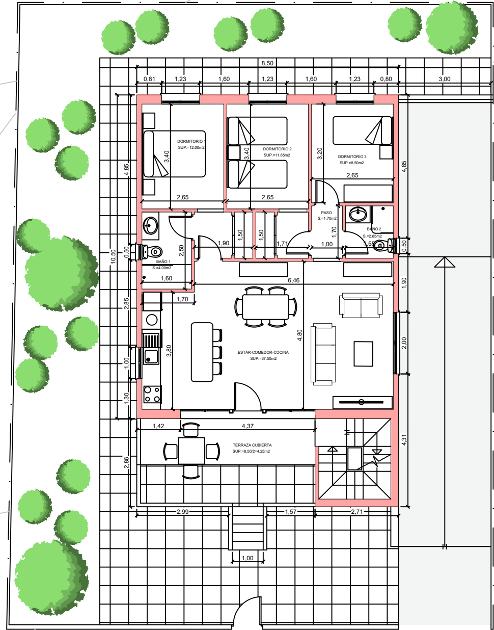
PLANTA BAJA
