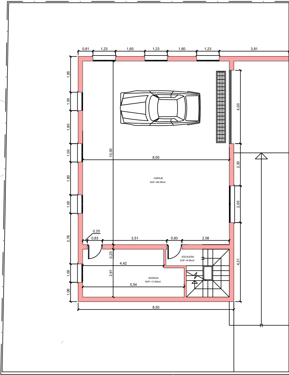
PLANTA SEMISOTANO
