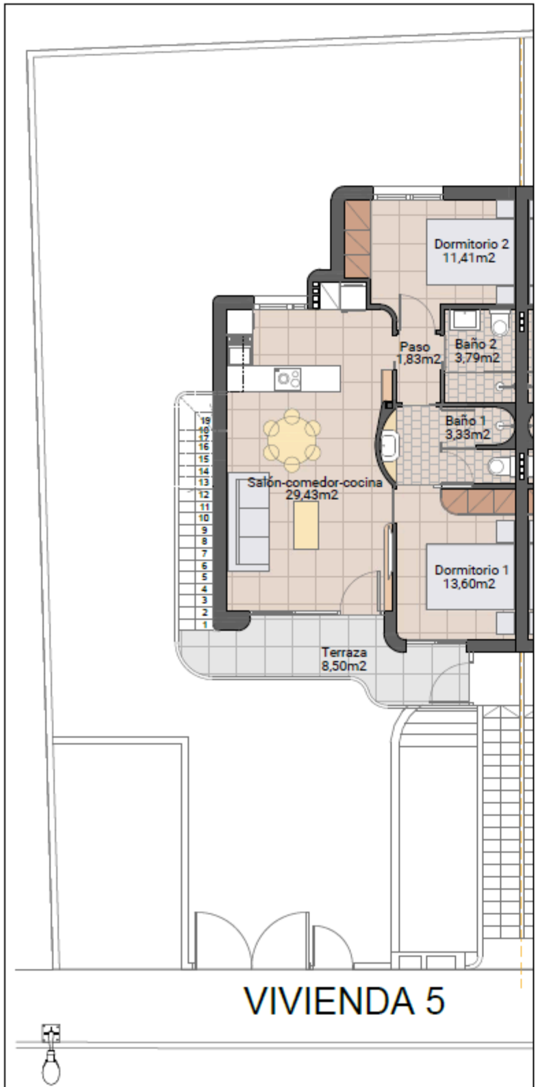
PLANTA PRIMERA
