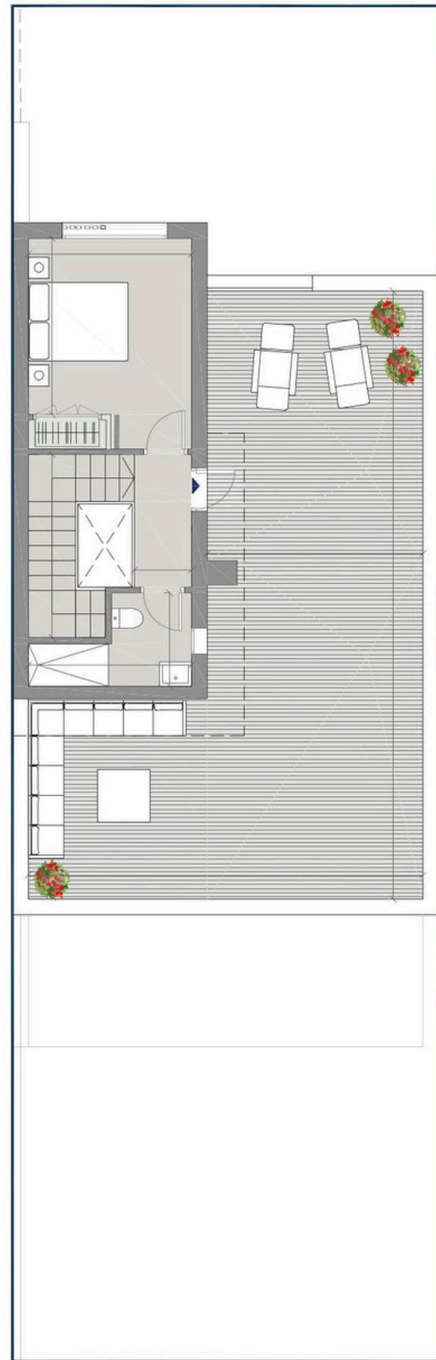
PLANTA ÁTICO
