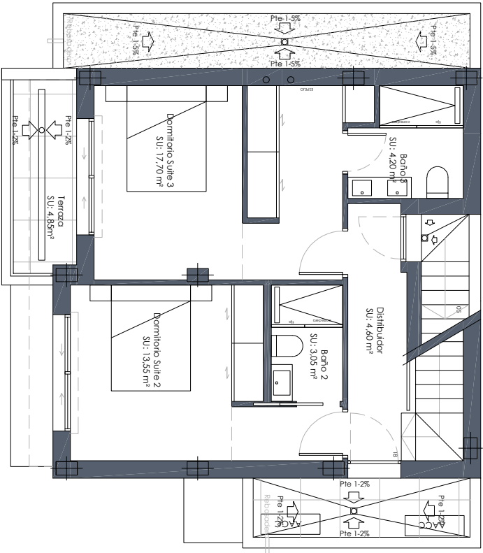
PLANTA PRIMERA
