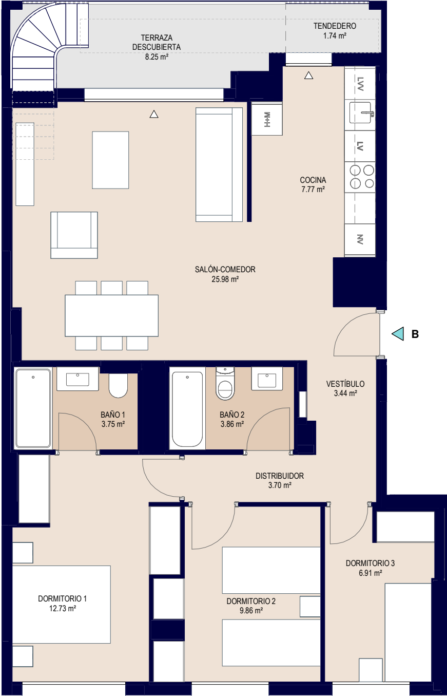
OPCION BASE 1 : 75
