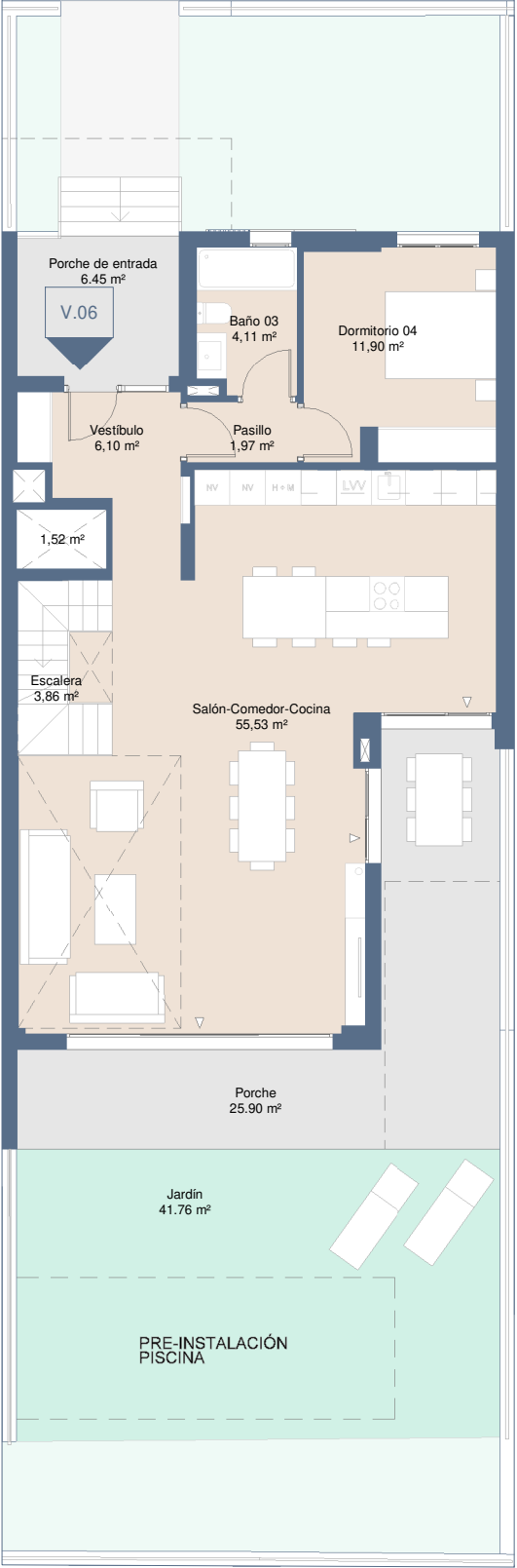
PLANTA BAJA COMPLETA
