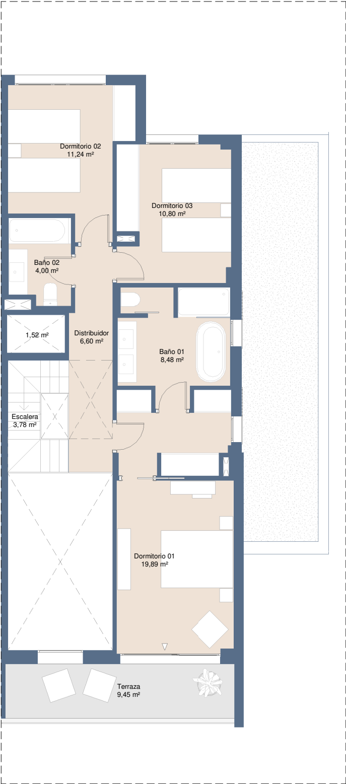
PLANTA PRIMERA
