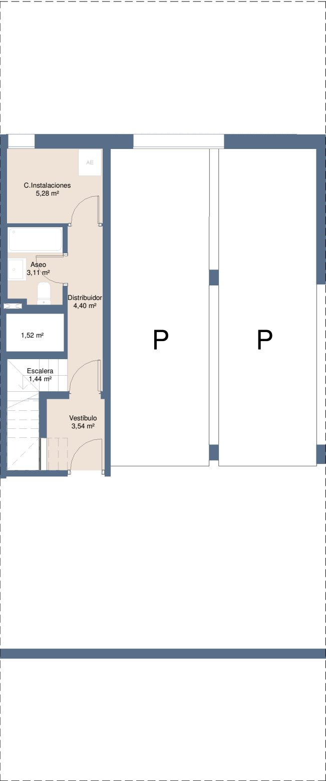
PLANTA SÓTANO
