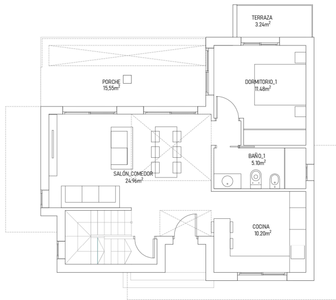
PLANTA BAJA OPCIÓN A
