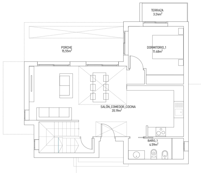
PLANTA BAJA OPCIÓN B
