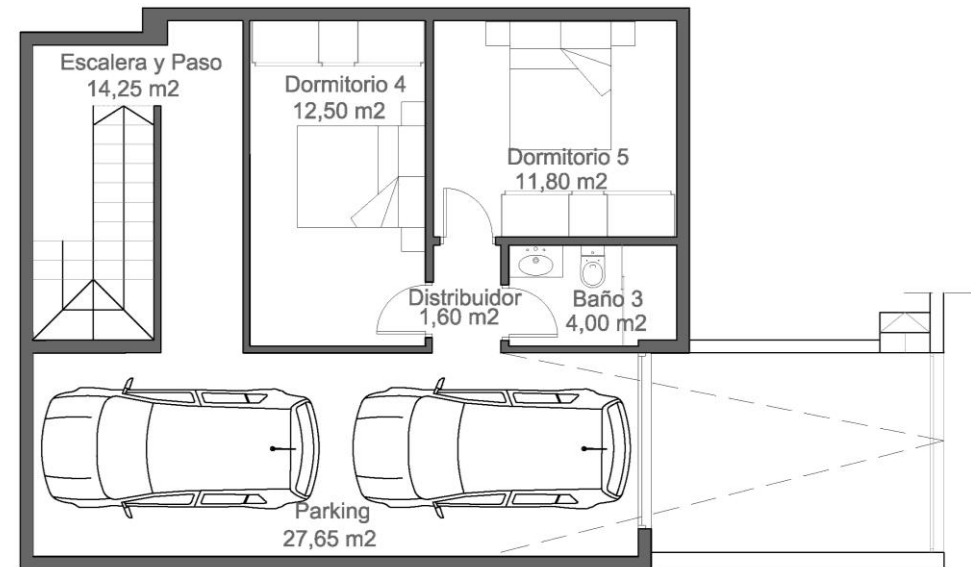
PLANTA SÓTANO
