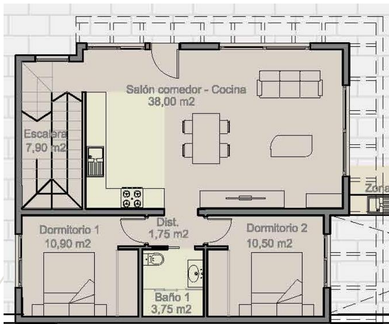
PLANTA BAJA
