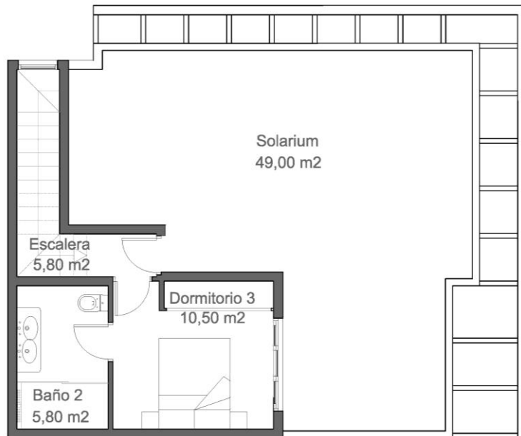
PLANTA PRIMERA
