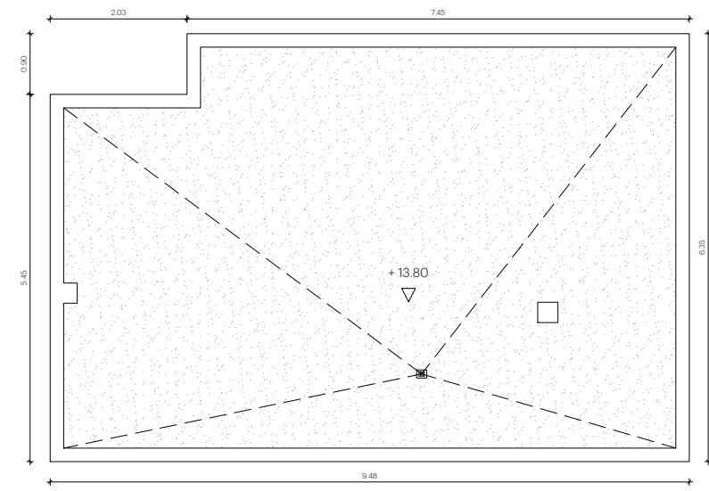
CUBIERTA TORREON
