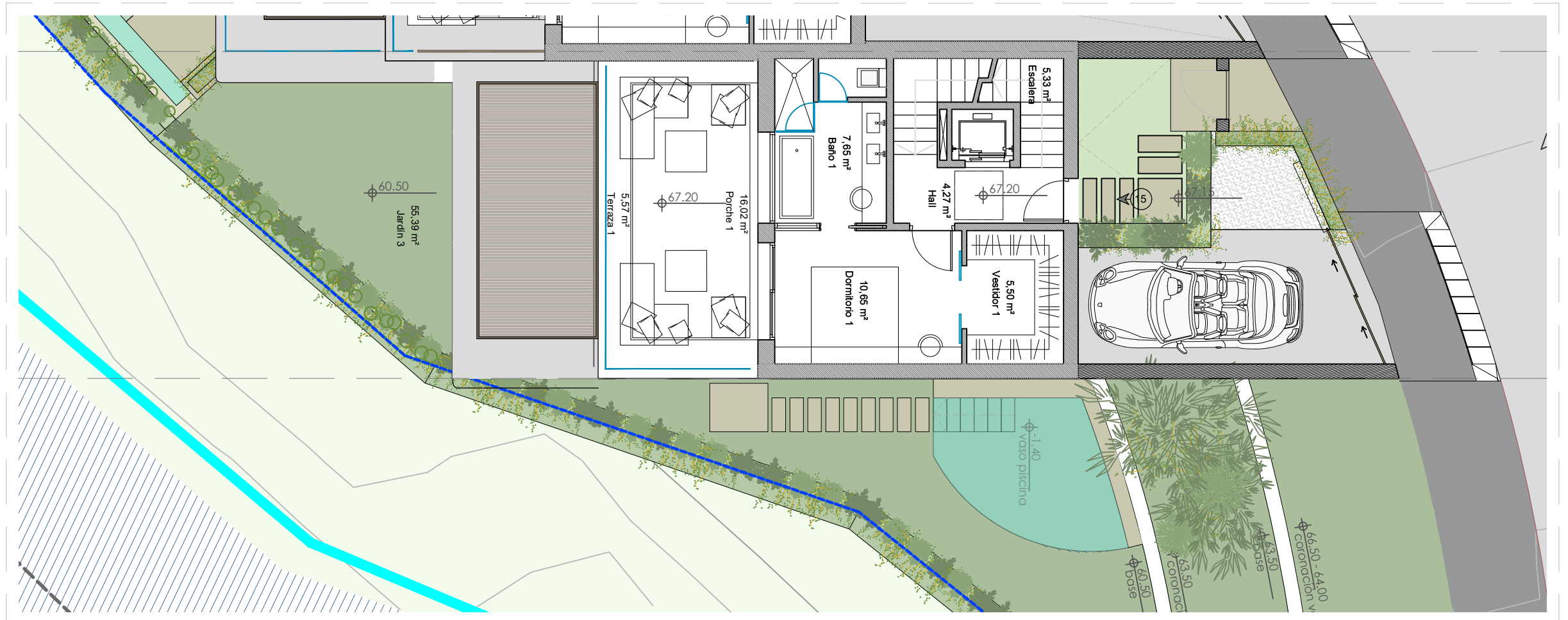
NIVEL 0
