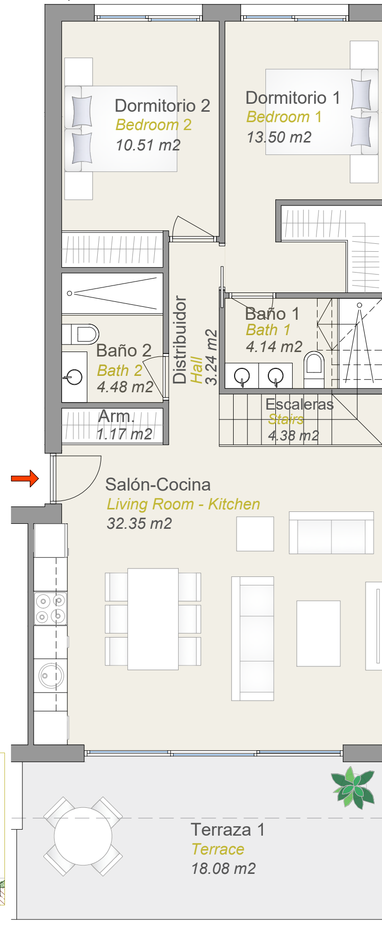
PLANTA PRINCIPAL
