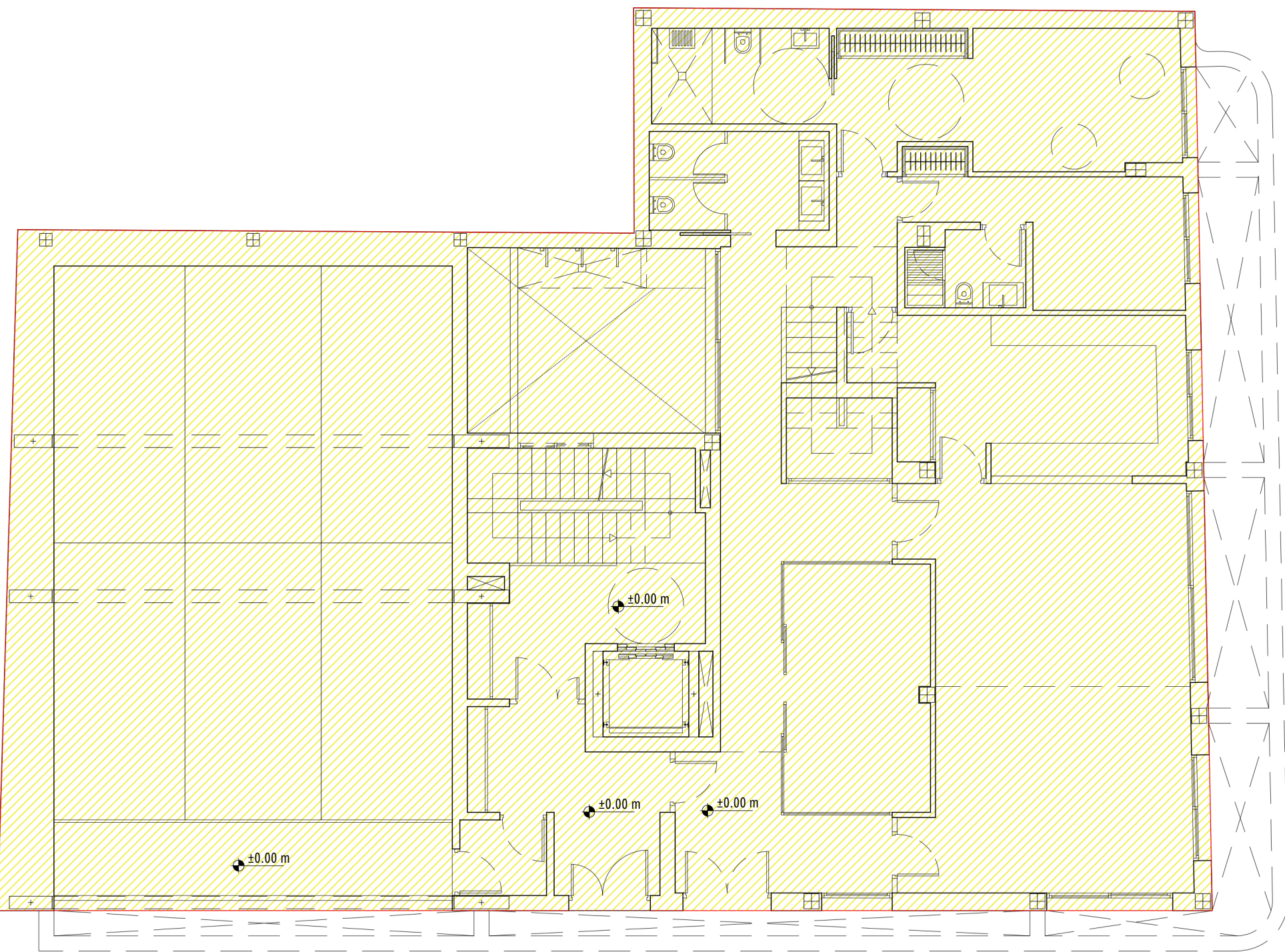
PLANTA BAJA
