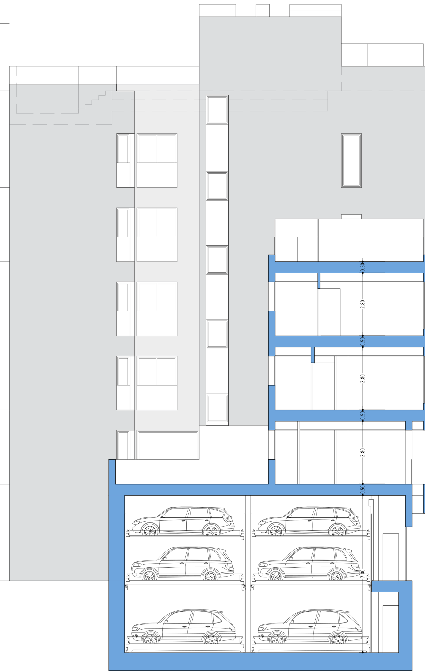
SECCIÓN D-D'
