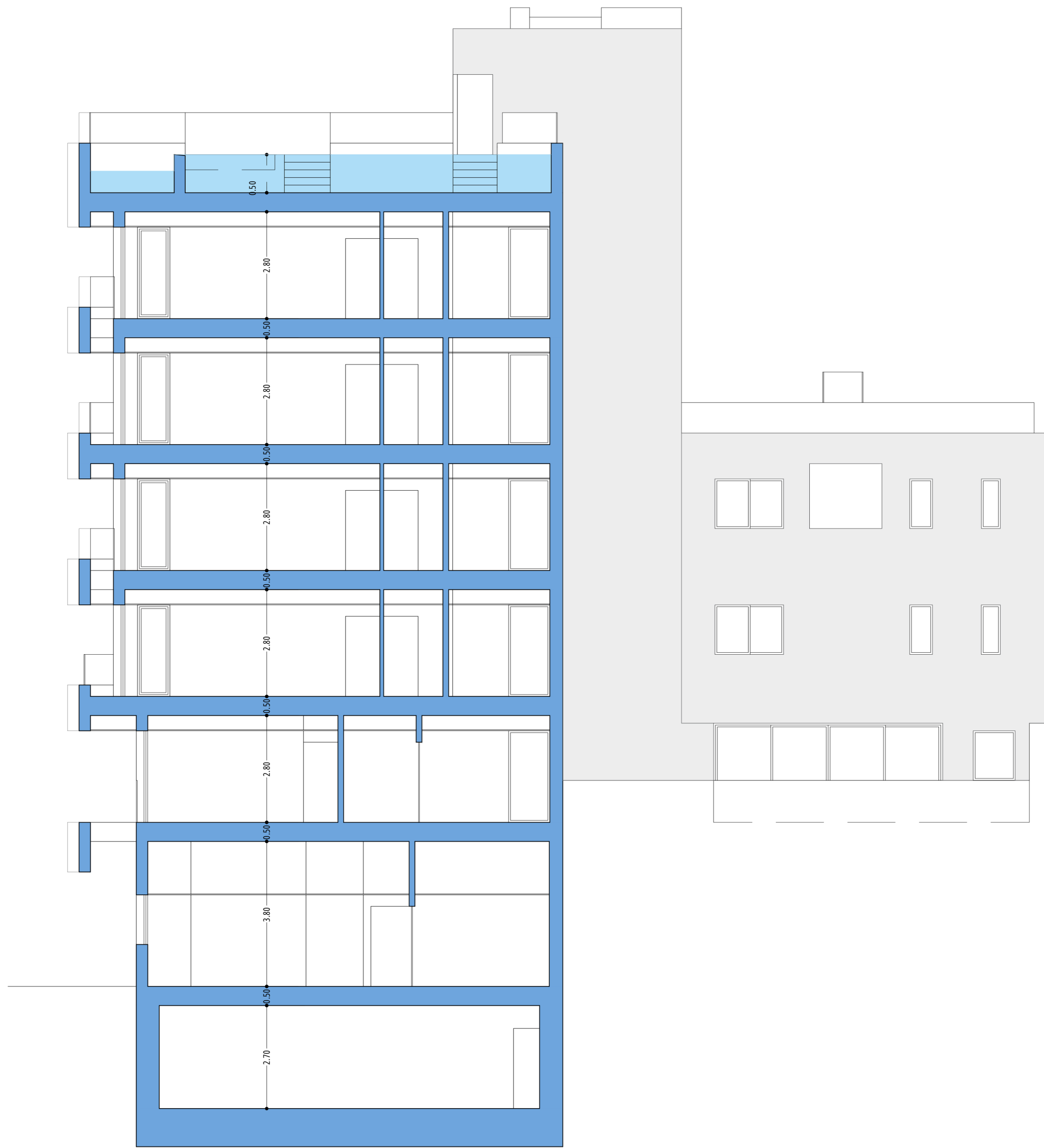
SECCIÓN C-C'
