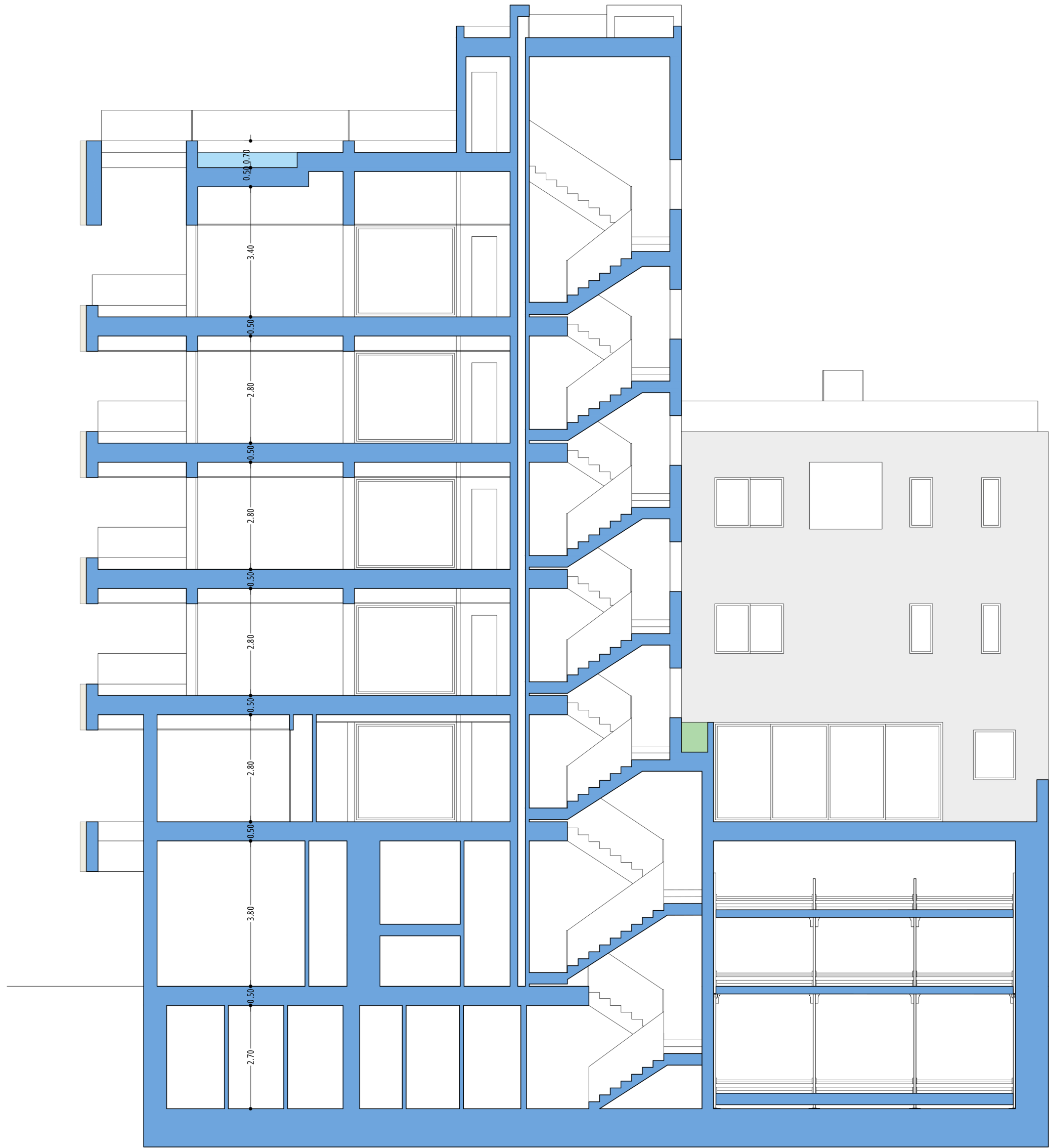
SECCIÓN A-A' 1:100
