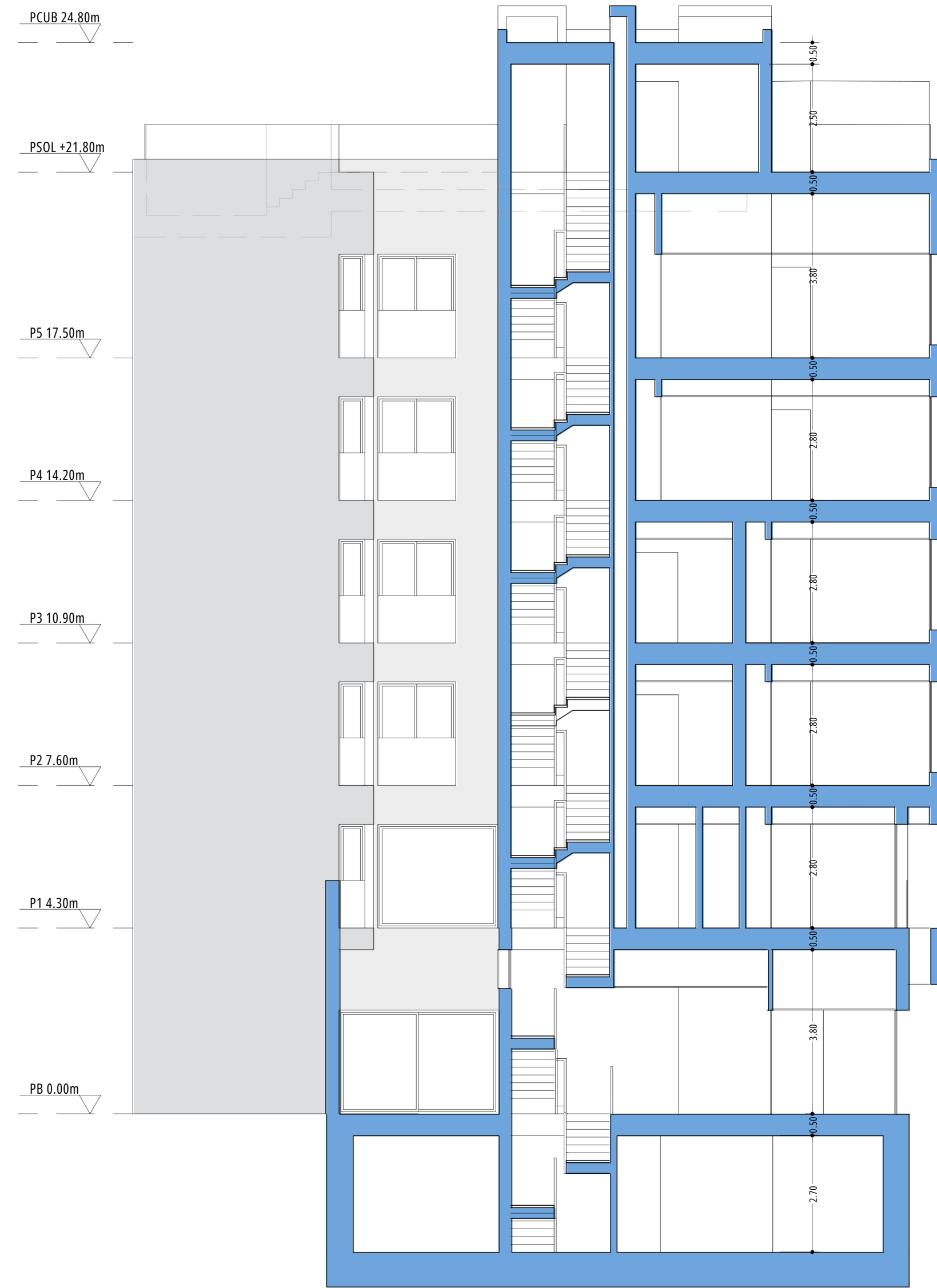
SECCIÓN B-B' 1:100
