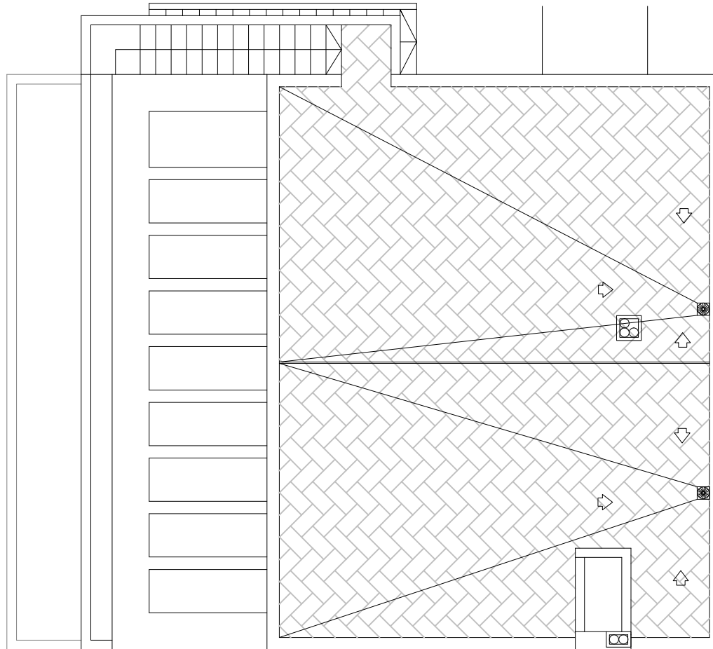
Planta Solarium
