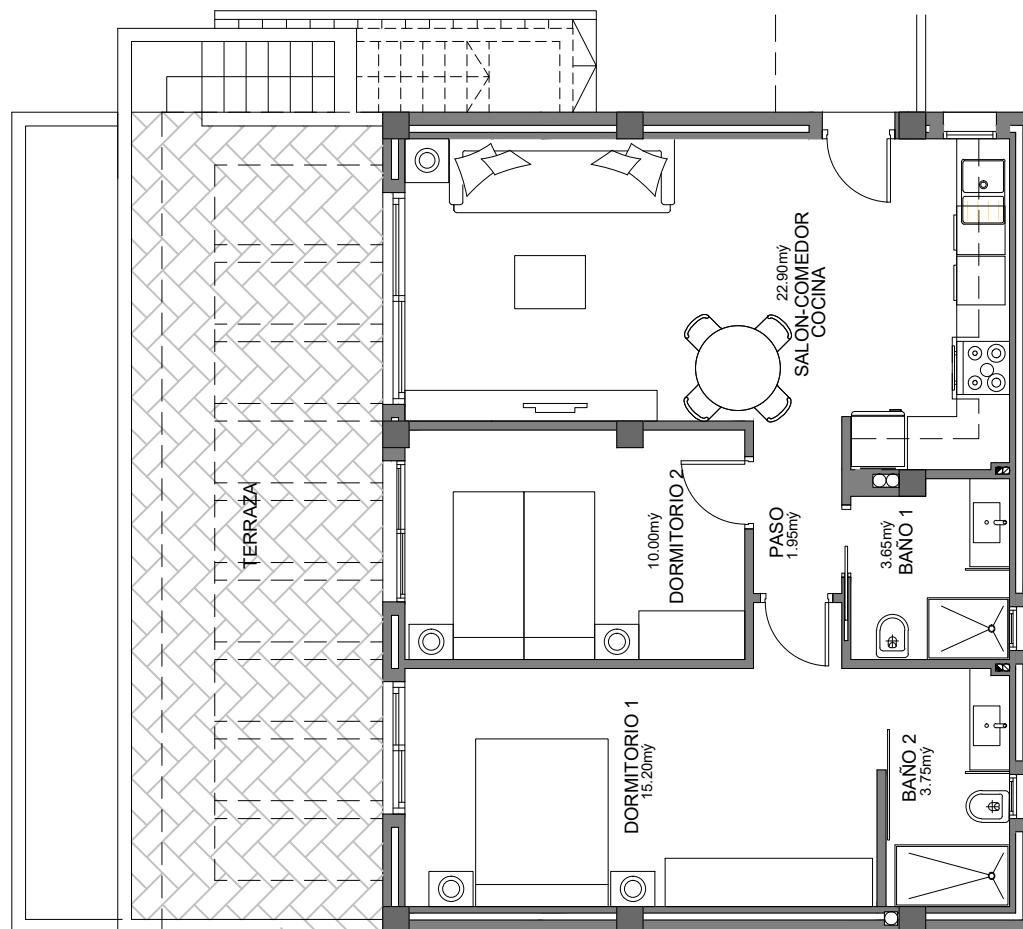
Planta Primera
