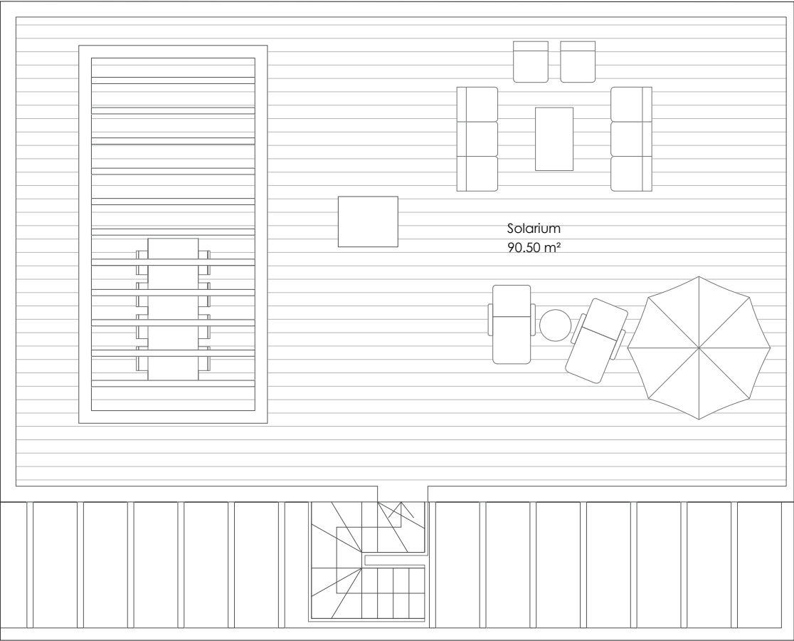
PLANTA SOLARIUM
