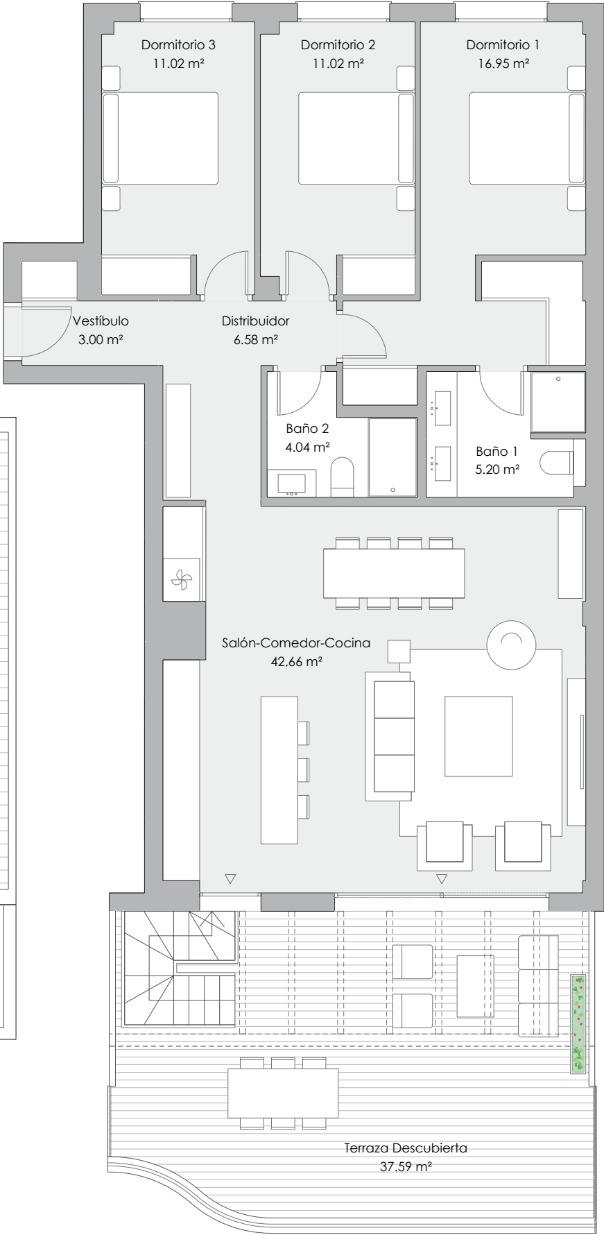
PLANTA SEGUNDA
