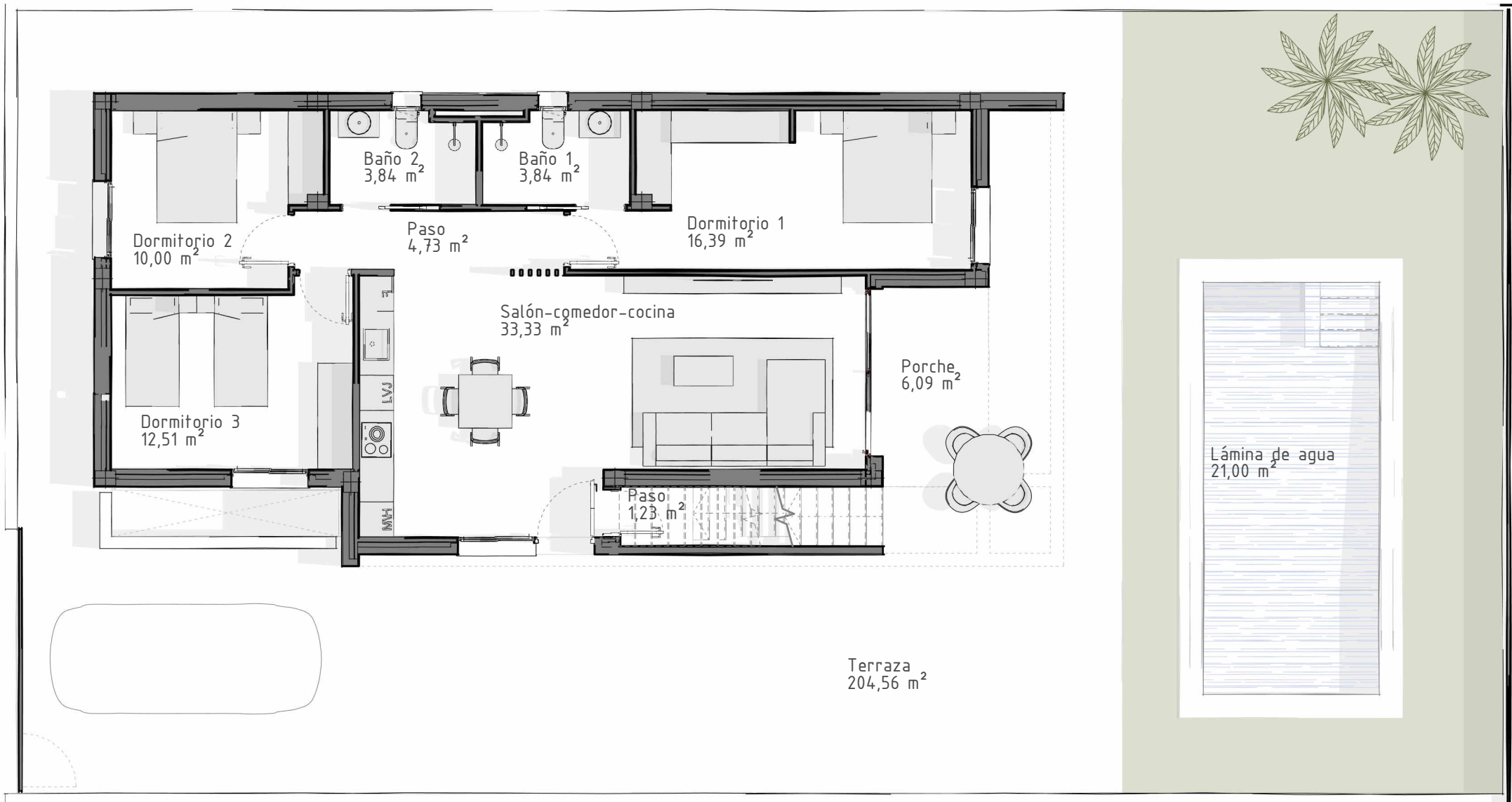
PLANTA BAJA
