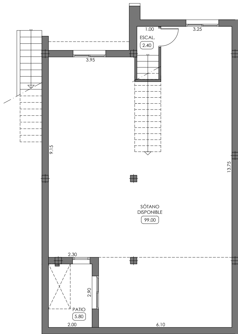
PLANTA SÓTANO
