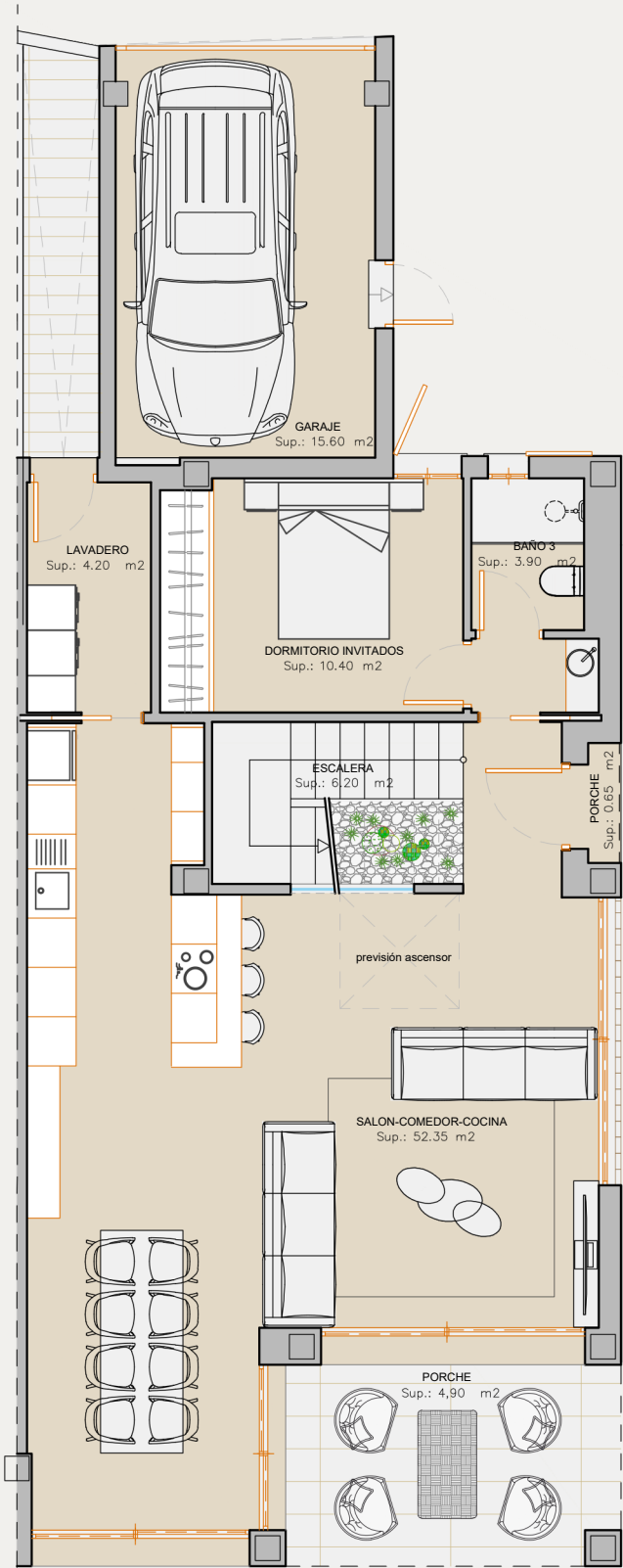
PLANTA BAJA
