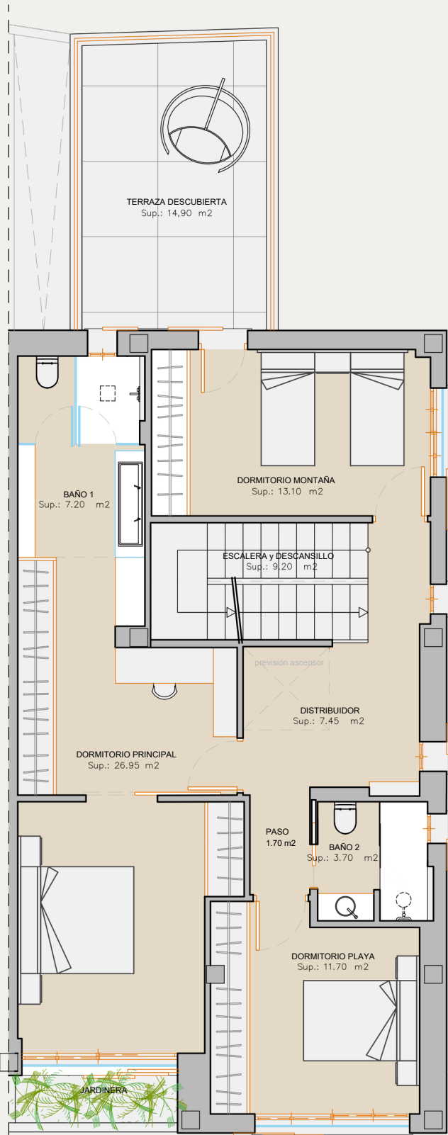
PLANTA PRIMERA
