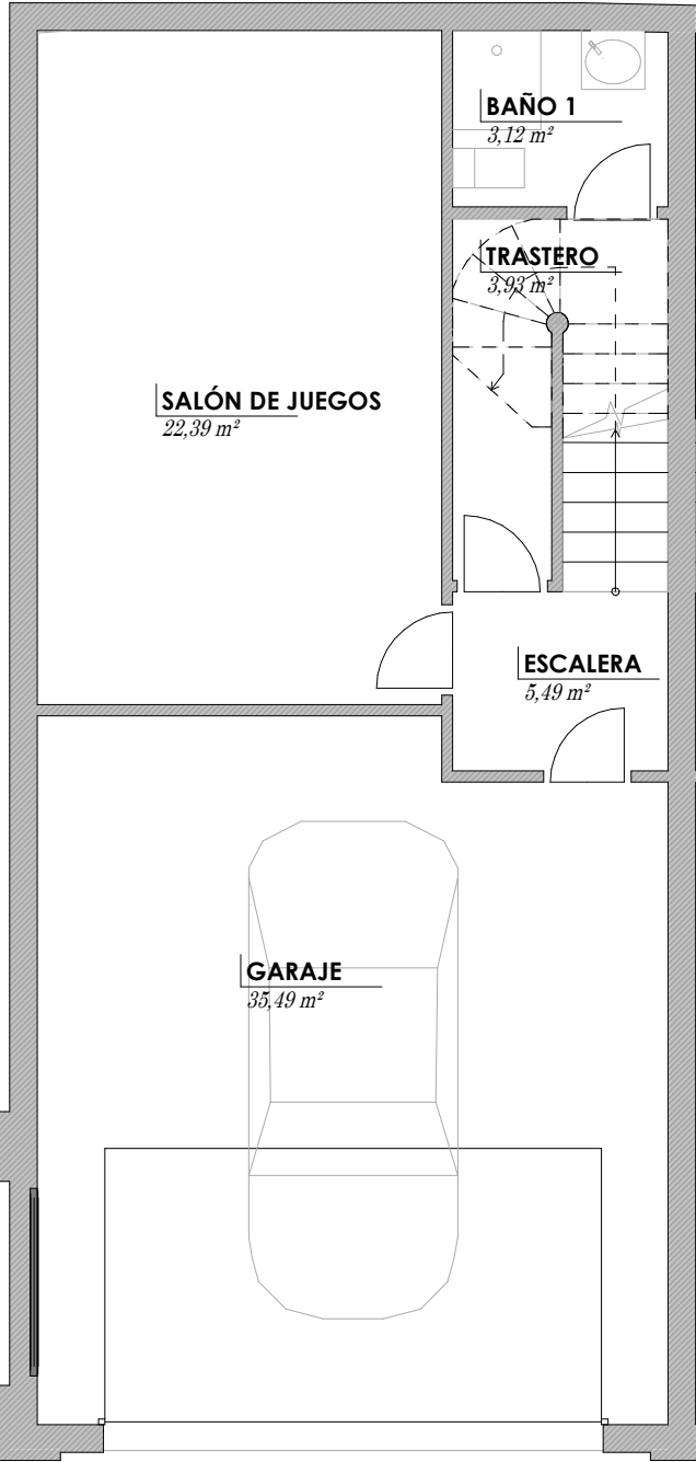
PLANTA SÓTANO
