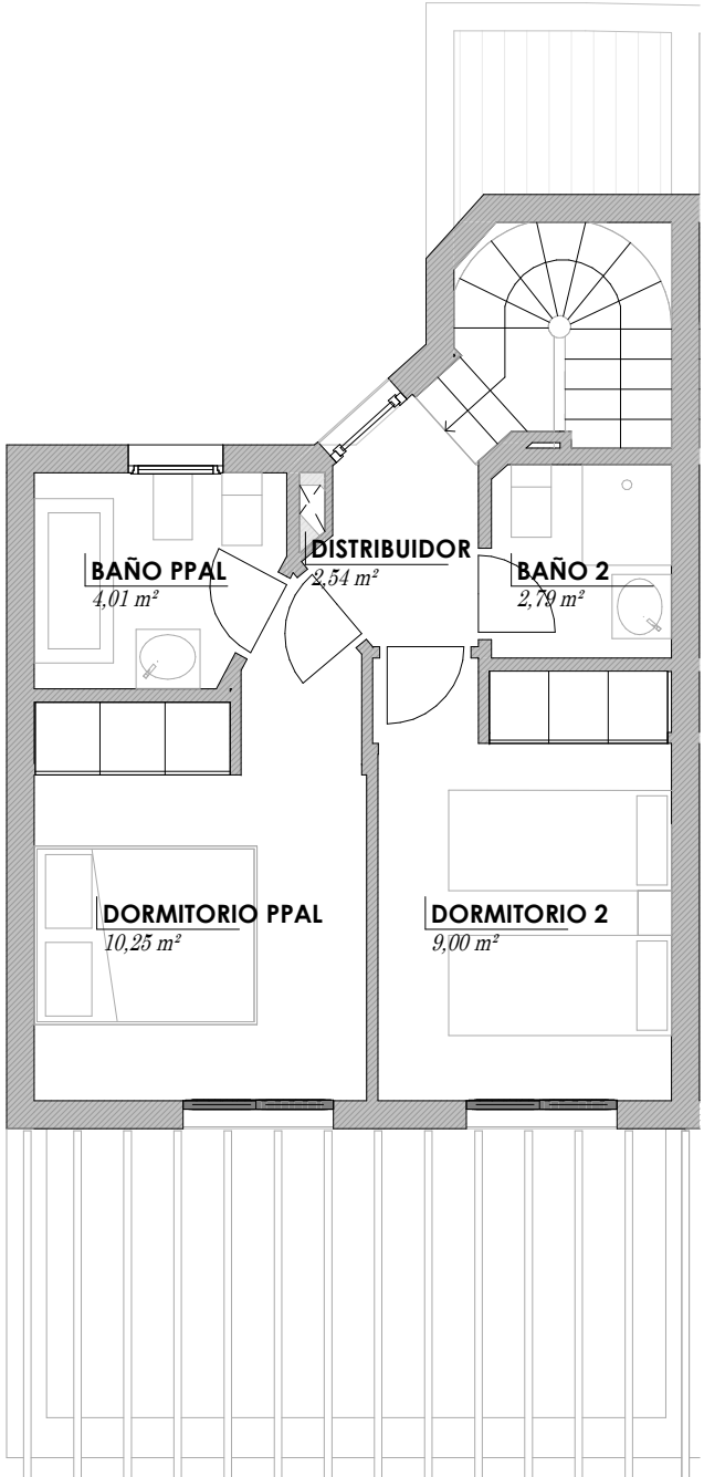
PLANTA PRIMERA
