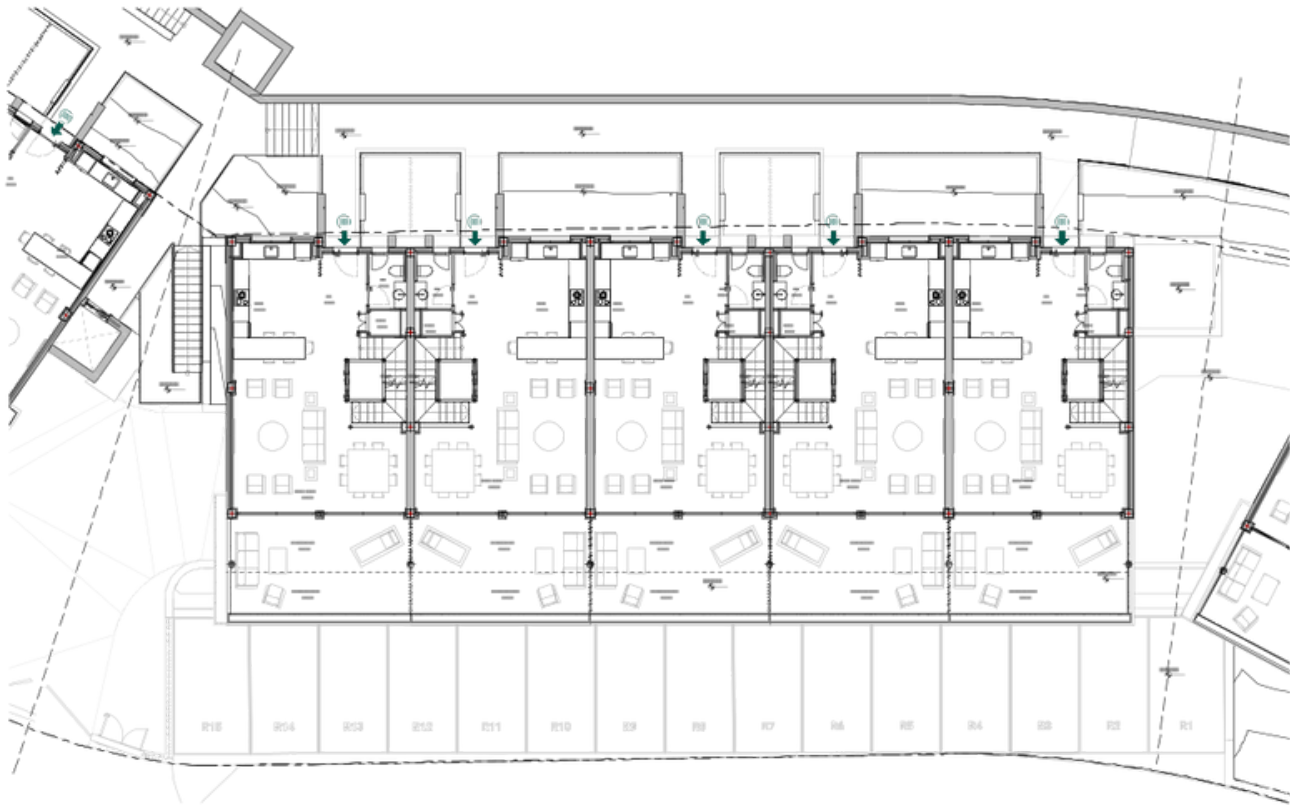
RESIDENCES 2 ACCESO 1:100
