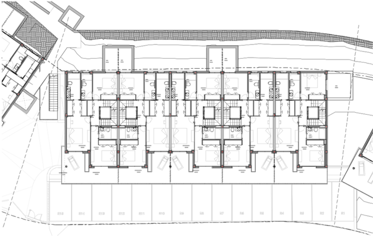
RESIDENCES 2 ACCESO 1:100
