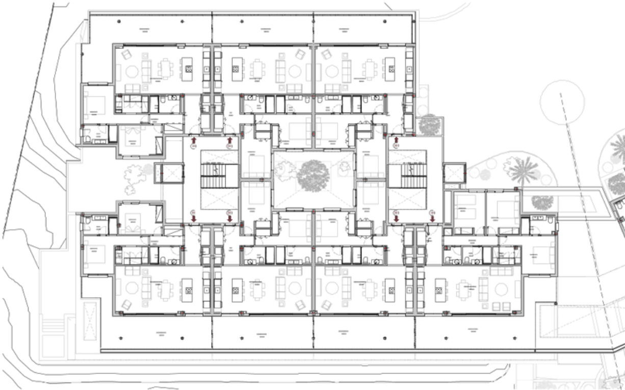
N.1 P1 SUITES 2 1:100
