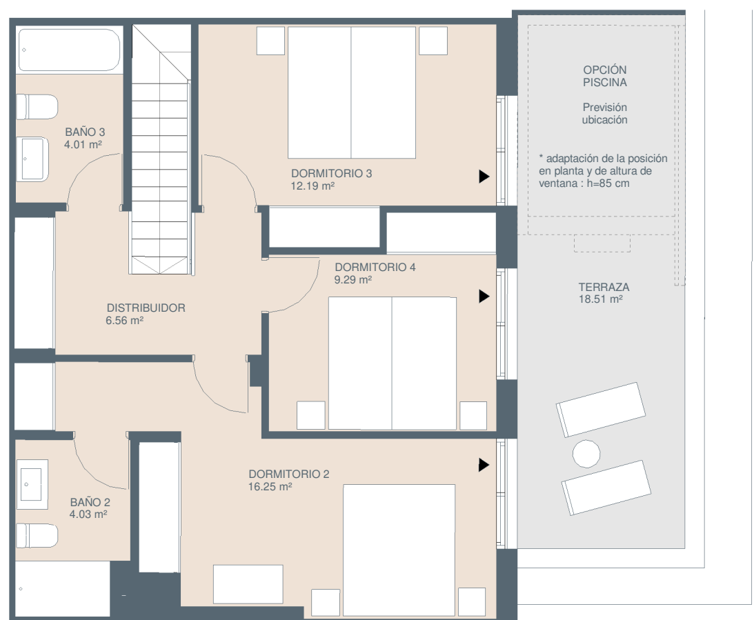
Planta bajo cubierta (nivel superior)
