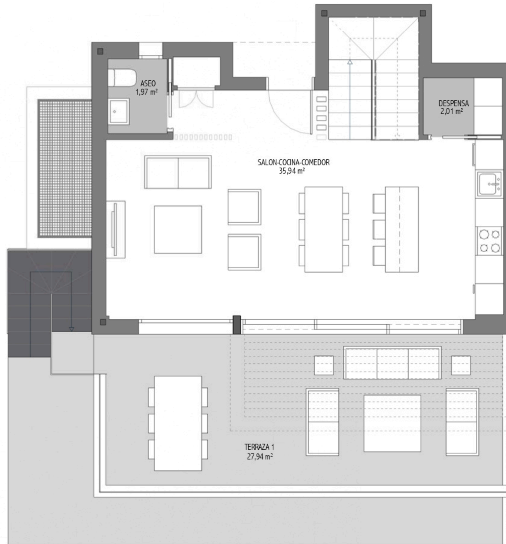
PLANTA ALTA 1 : 75
