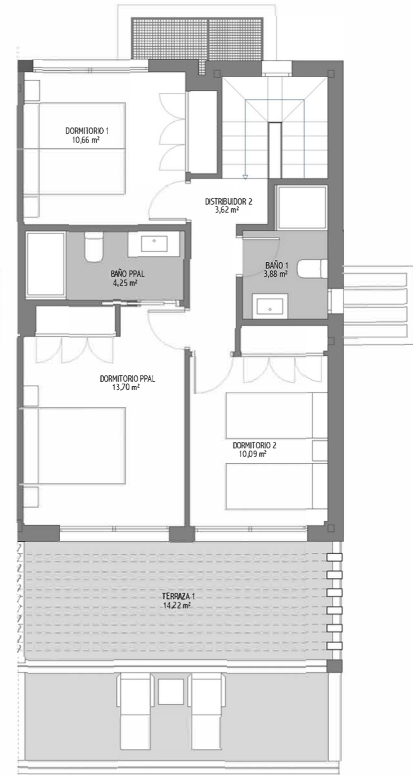
PLANTA ALTA 1:75
