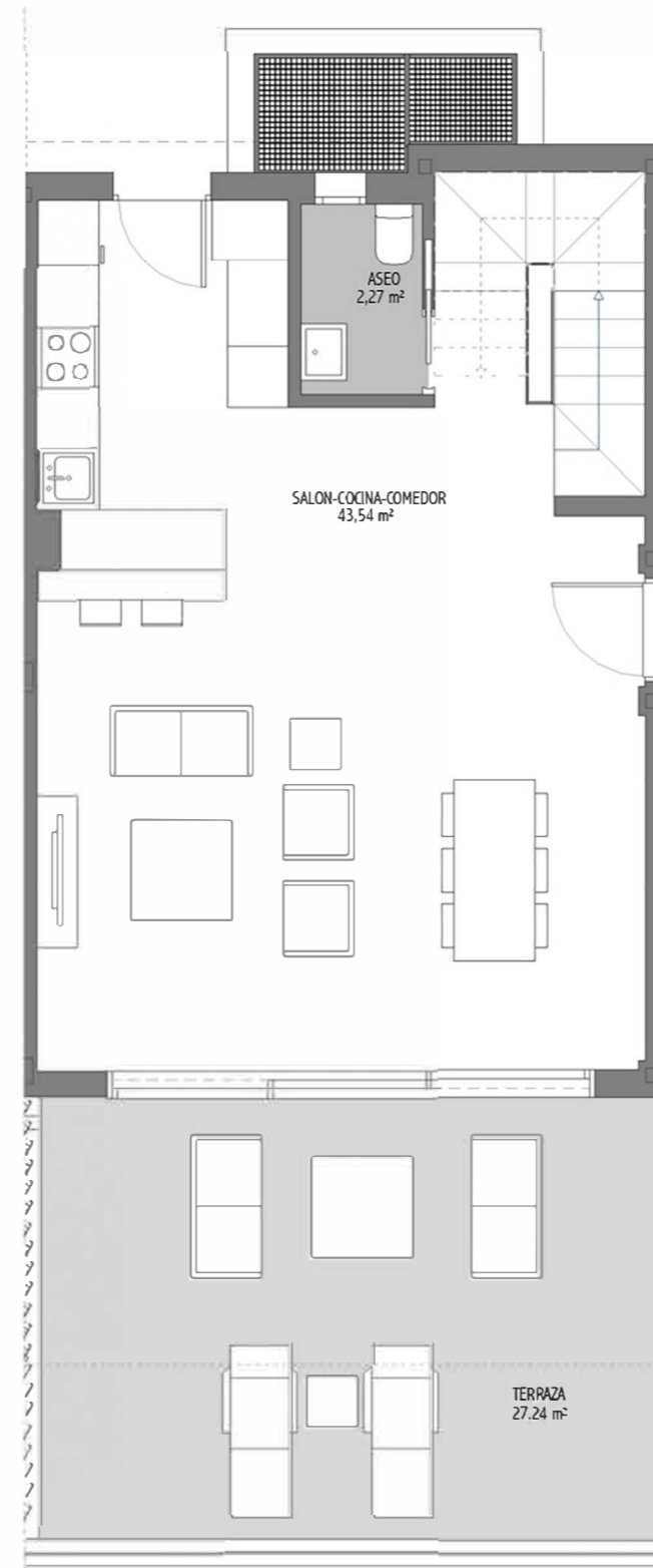
PLANTA BAJA 1:75
