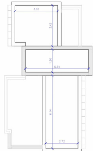
Planta Cubiertas
