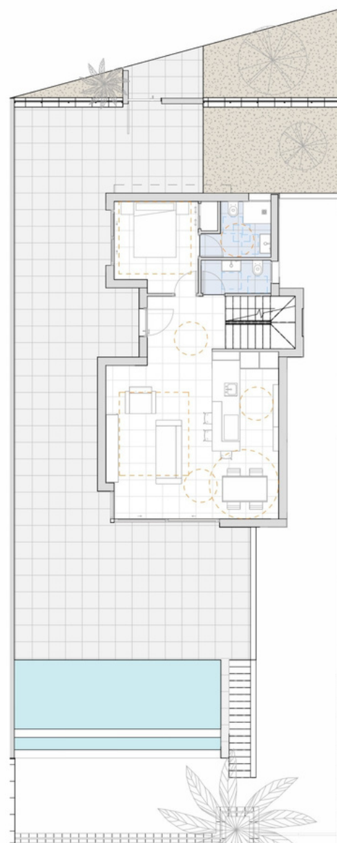
Planta Baja
