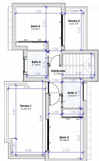
Planta Primera
