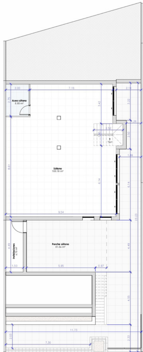
Planta Sótano
