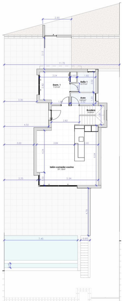
Planta Baja
