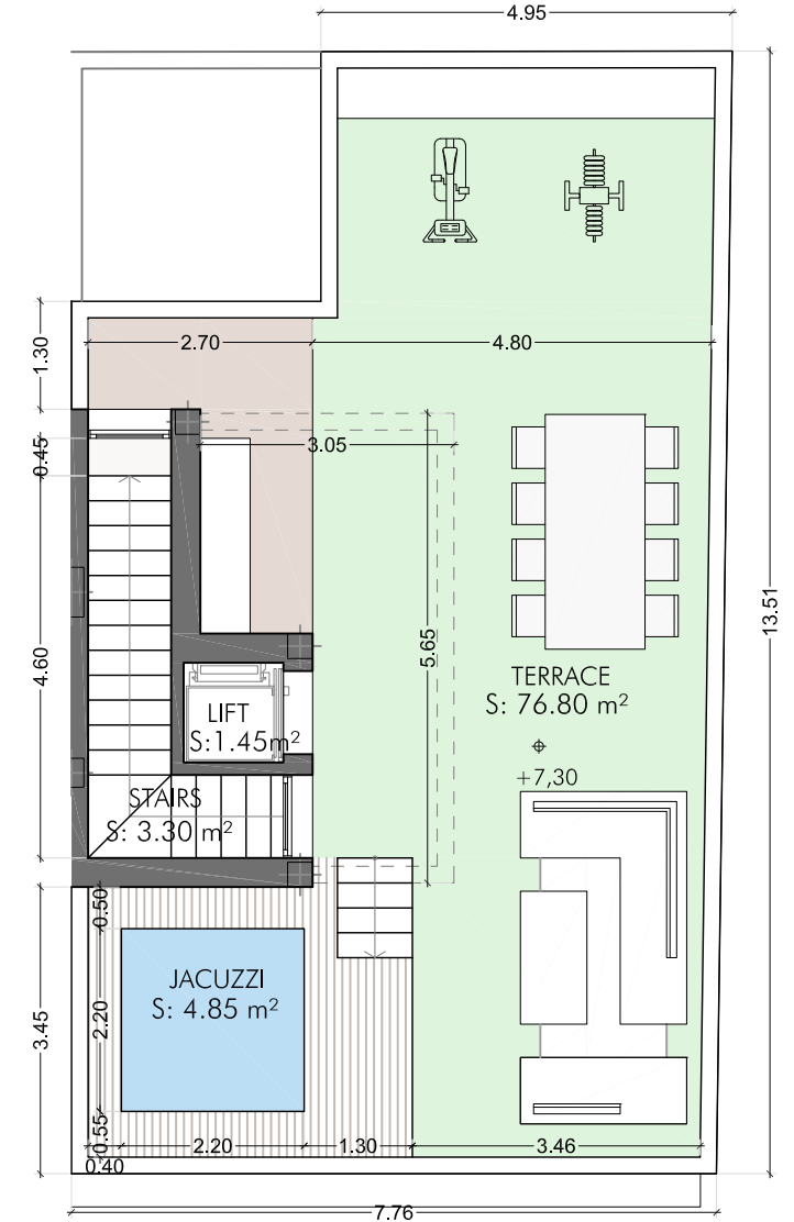
Solarium
