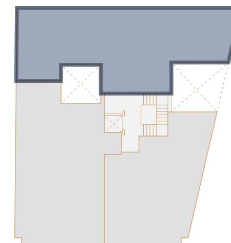
PLANTA 2º - 3º Puerta A
