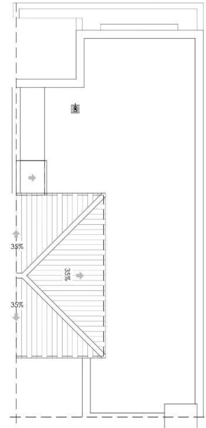
PLANTA DE CUBIERTA
