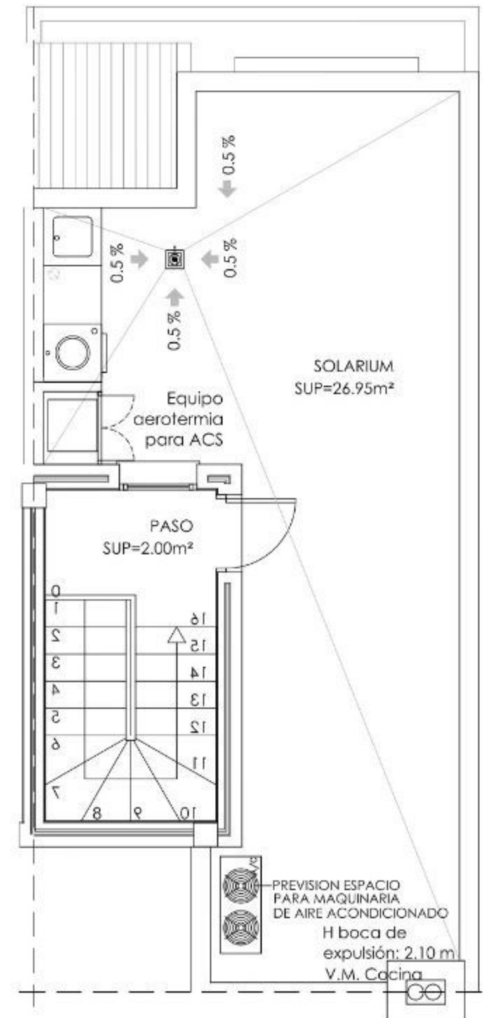
PLANTA TRASTERO
