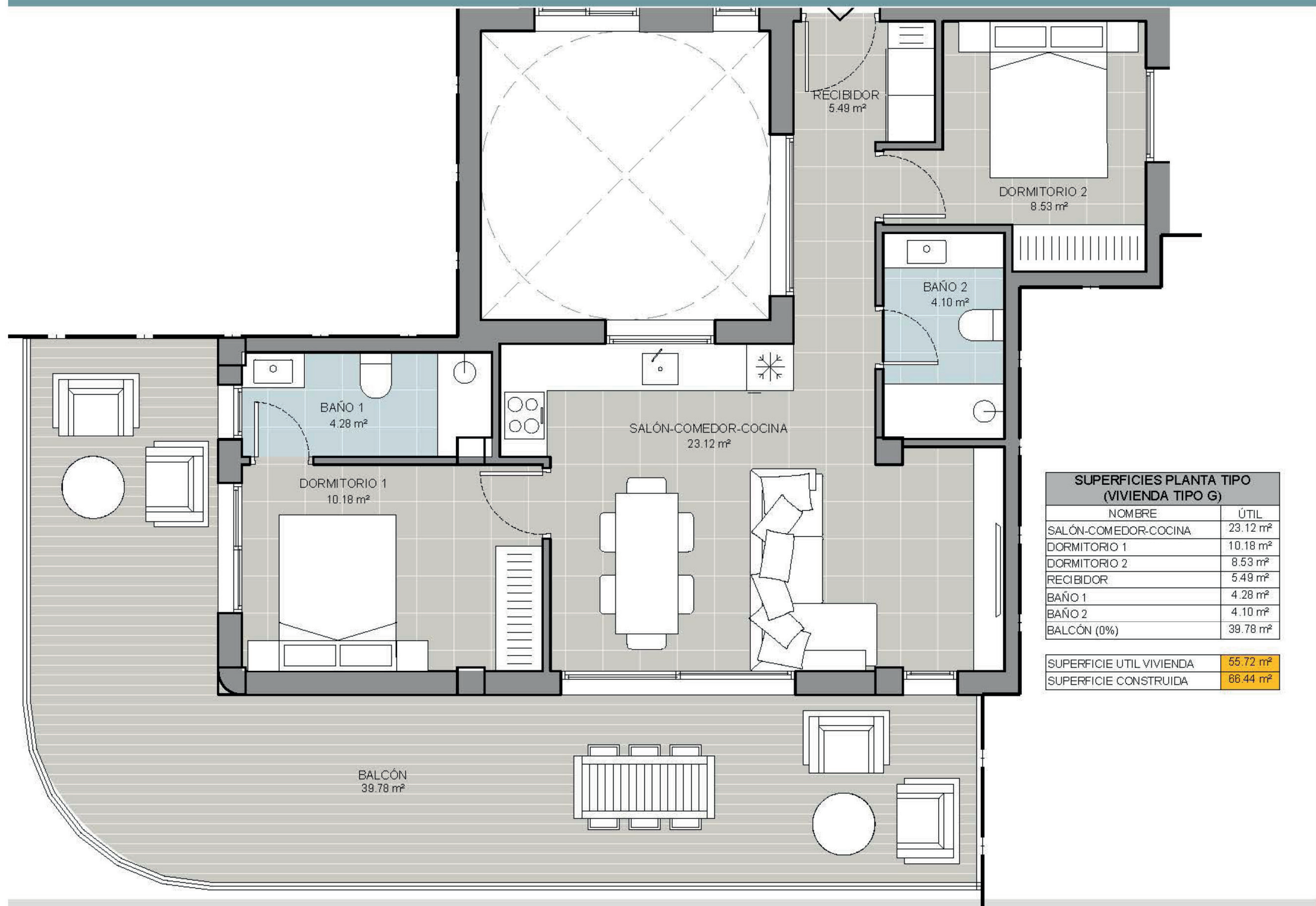
PLANTA 5 - ÁTICO G
