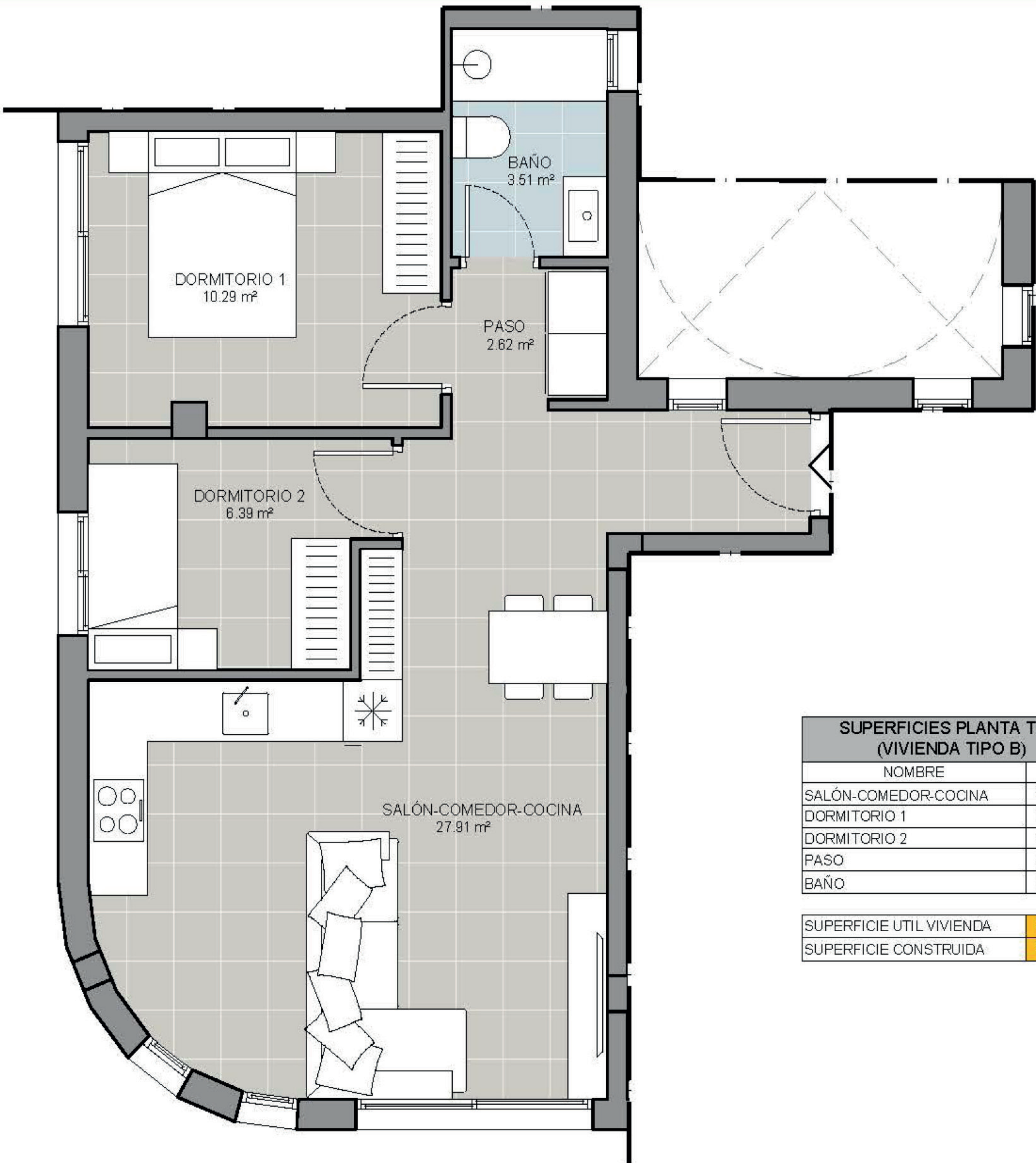
PLANTA 2 - VIVIENDA B
