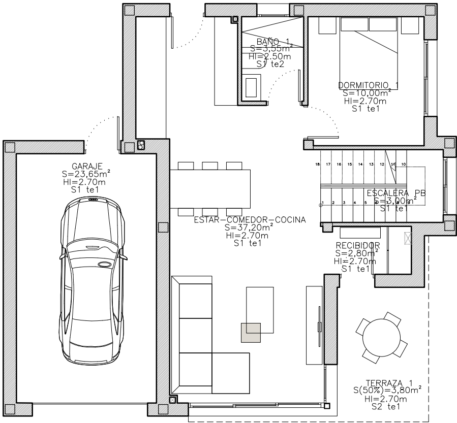
PLANTA BAJA
