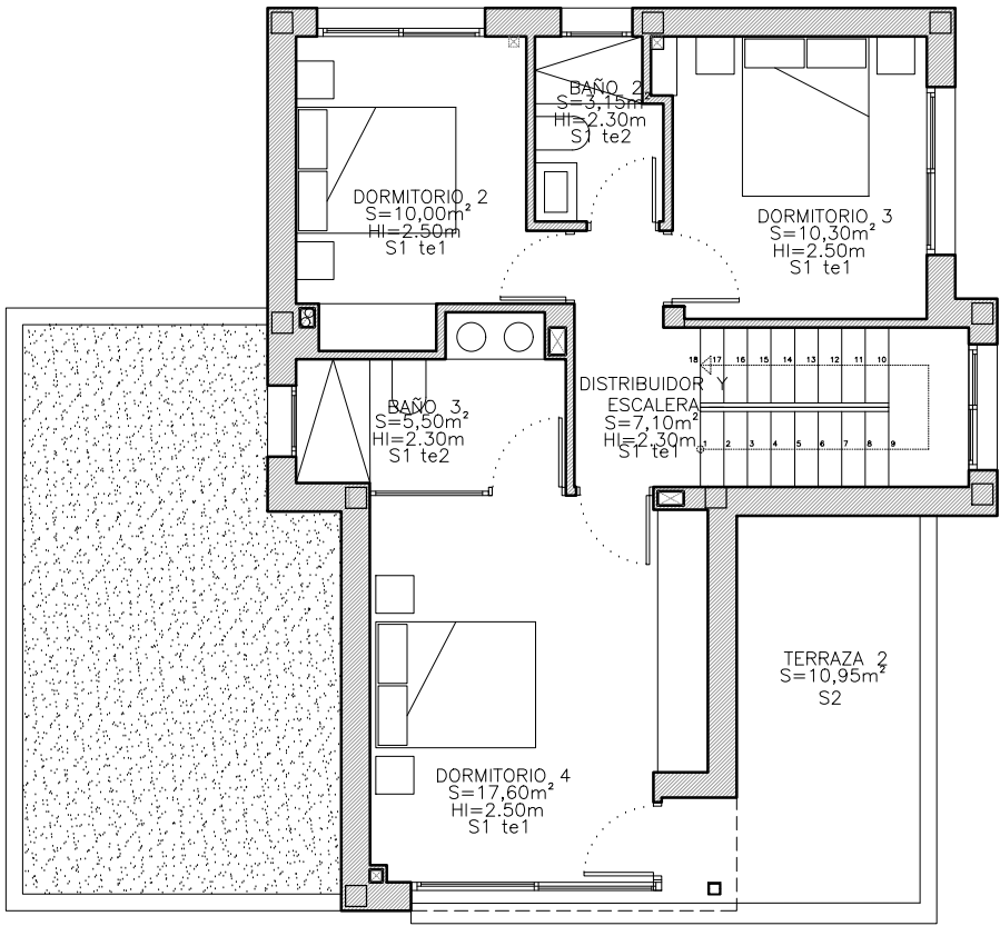
PLANTA PRIMERA
