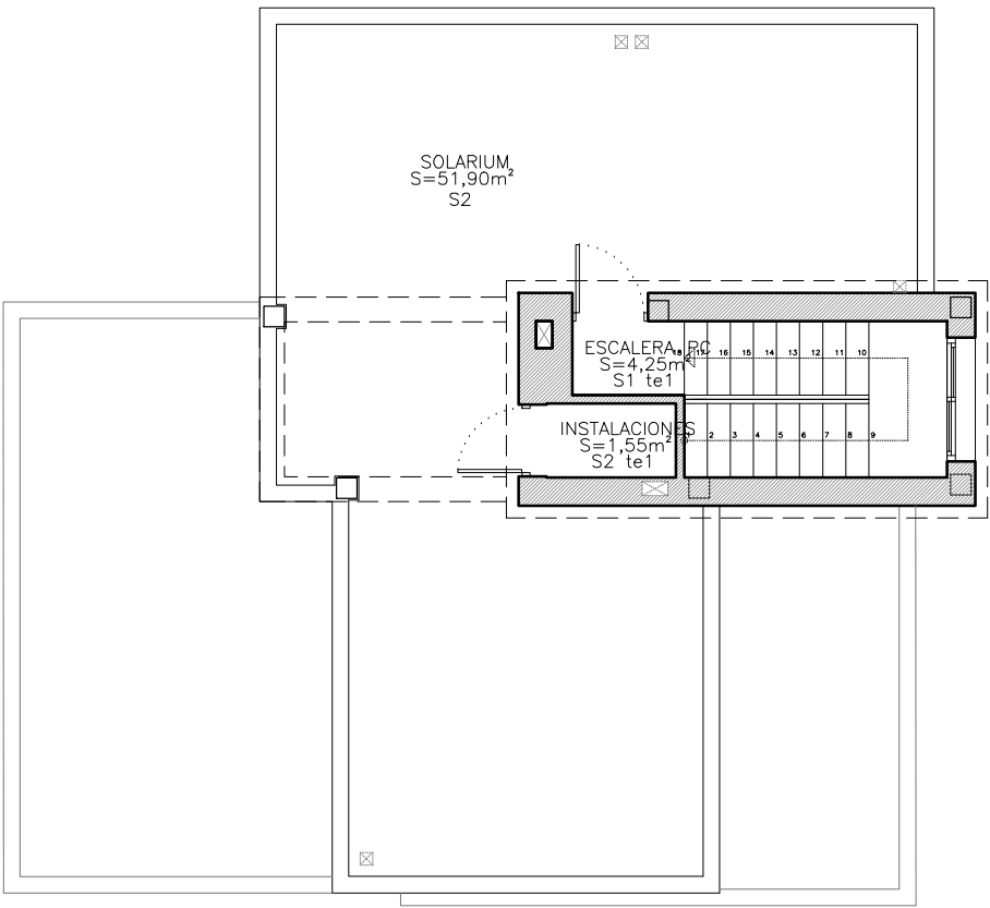
PLANTA SOLARIUM
