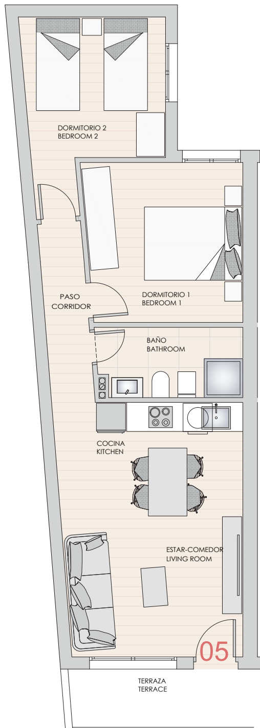
PLANTA PISO
