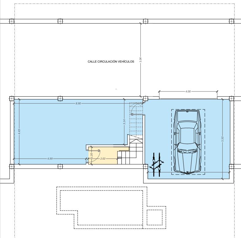
PLANTA SOTANO
