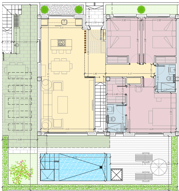
PLANTA BAJA
