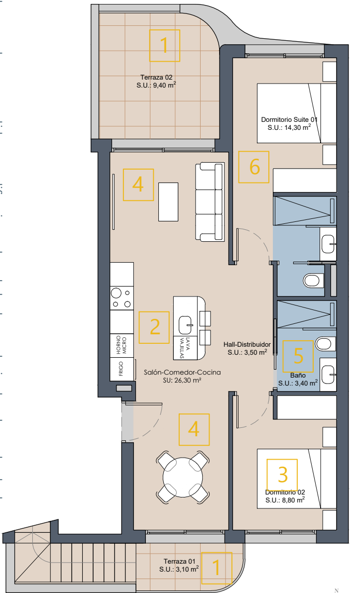
PLANTA SEGUNDA
