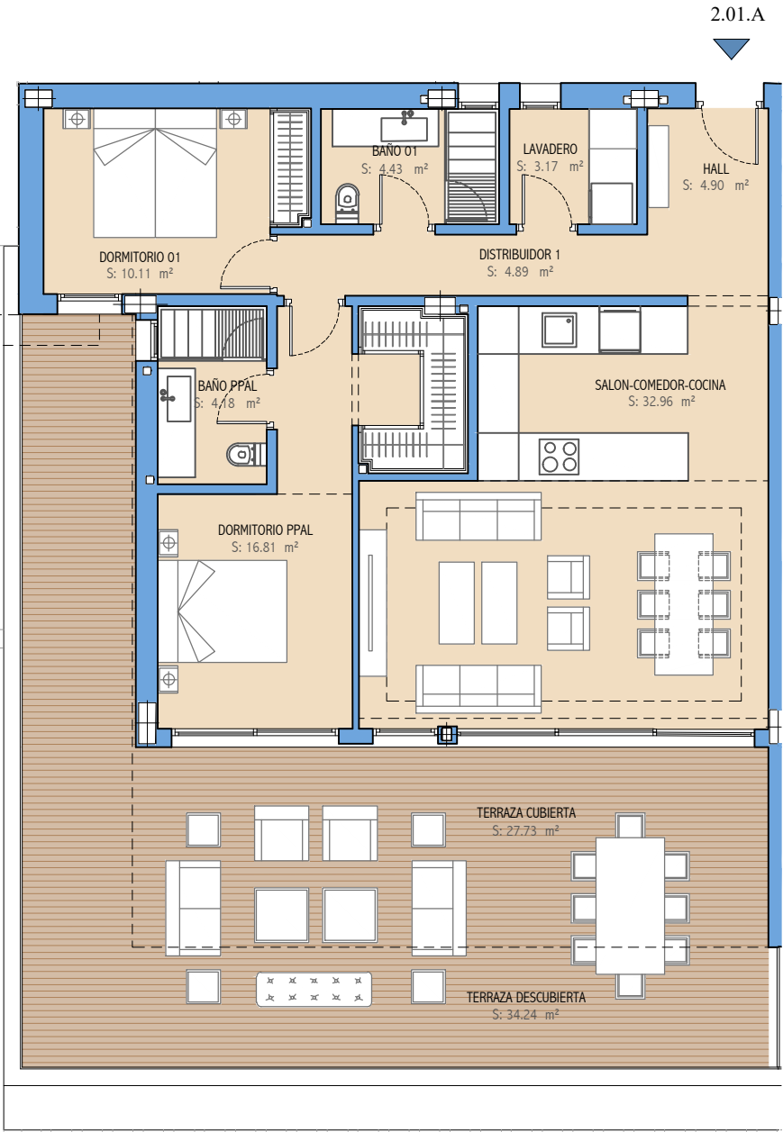
PLANTA PRIMERA
