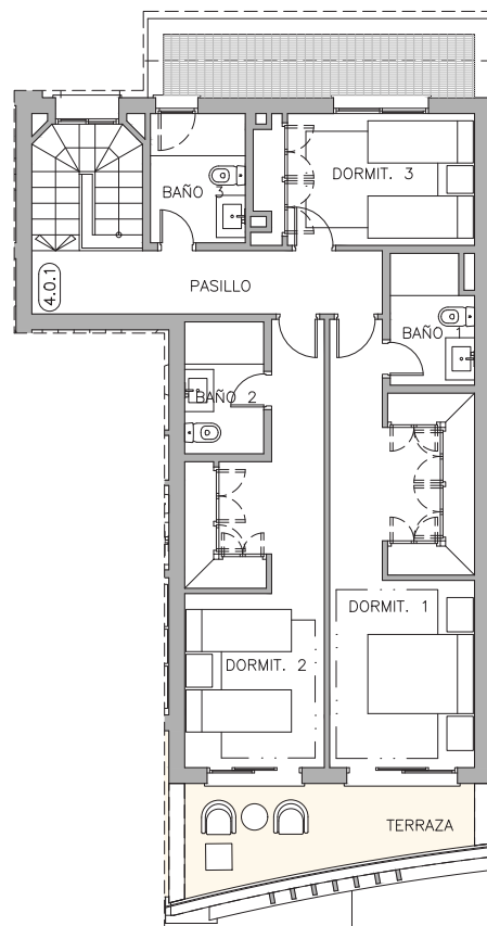
PLANTA PRIMERA
