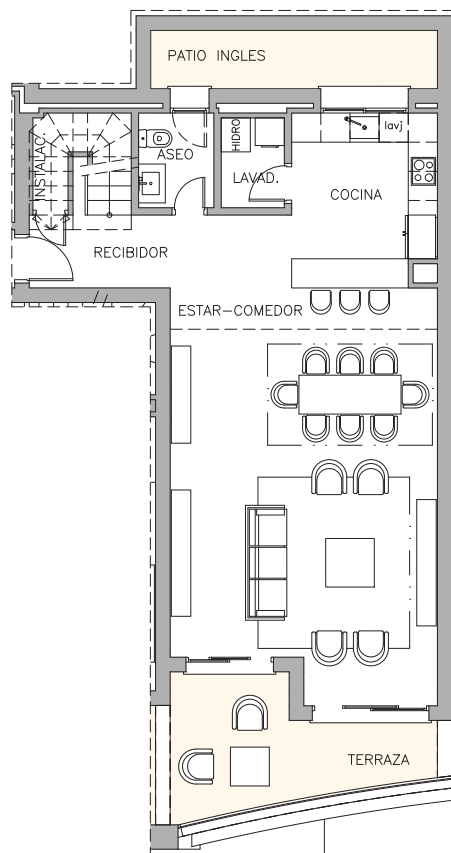
PLANTA 0
