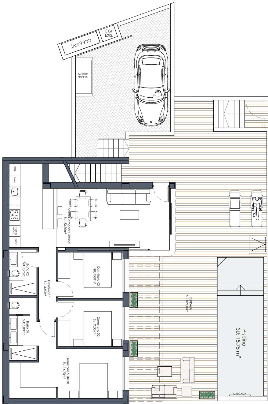
PLANTA BAJA
