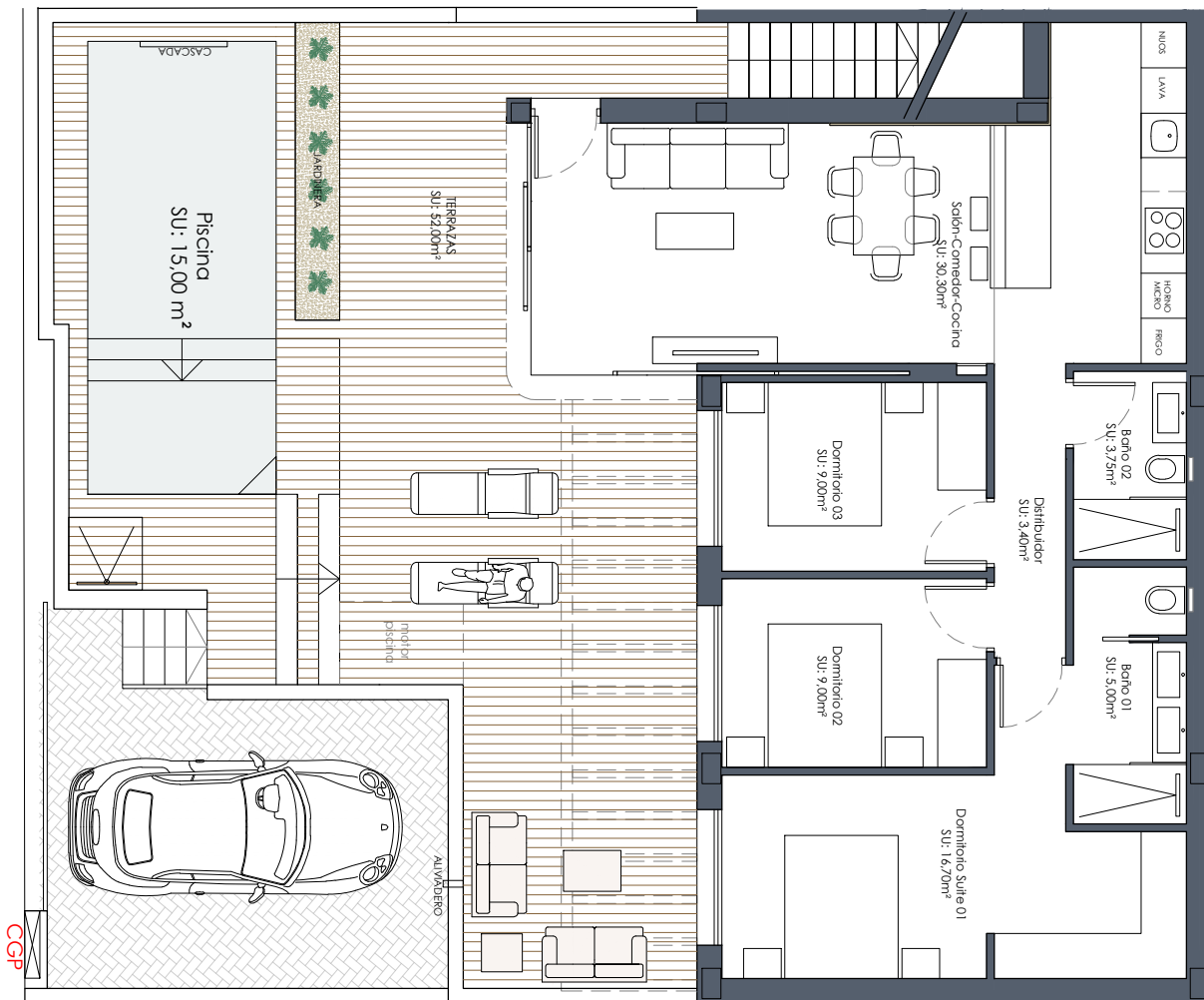
PLANTA BAJA
