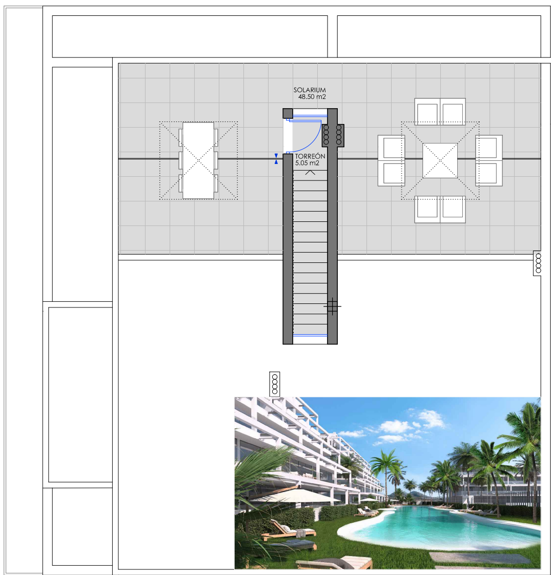
PLANTA SOLARIUM
