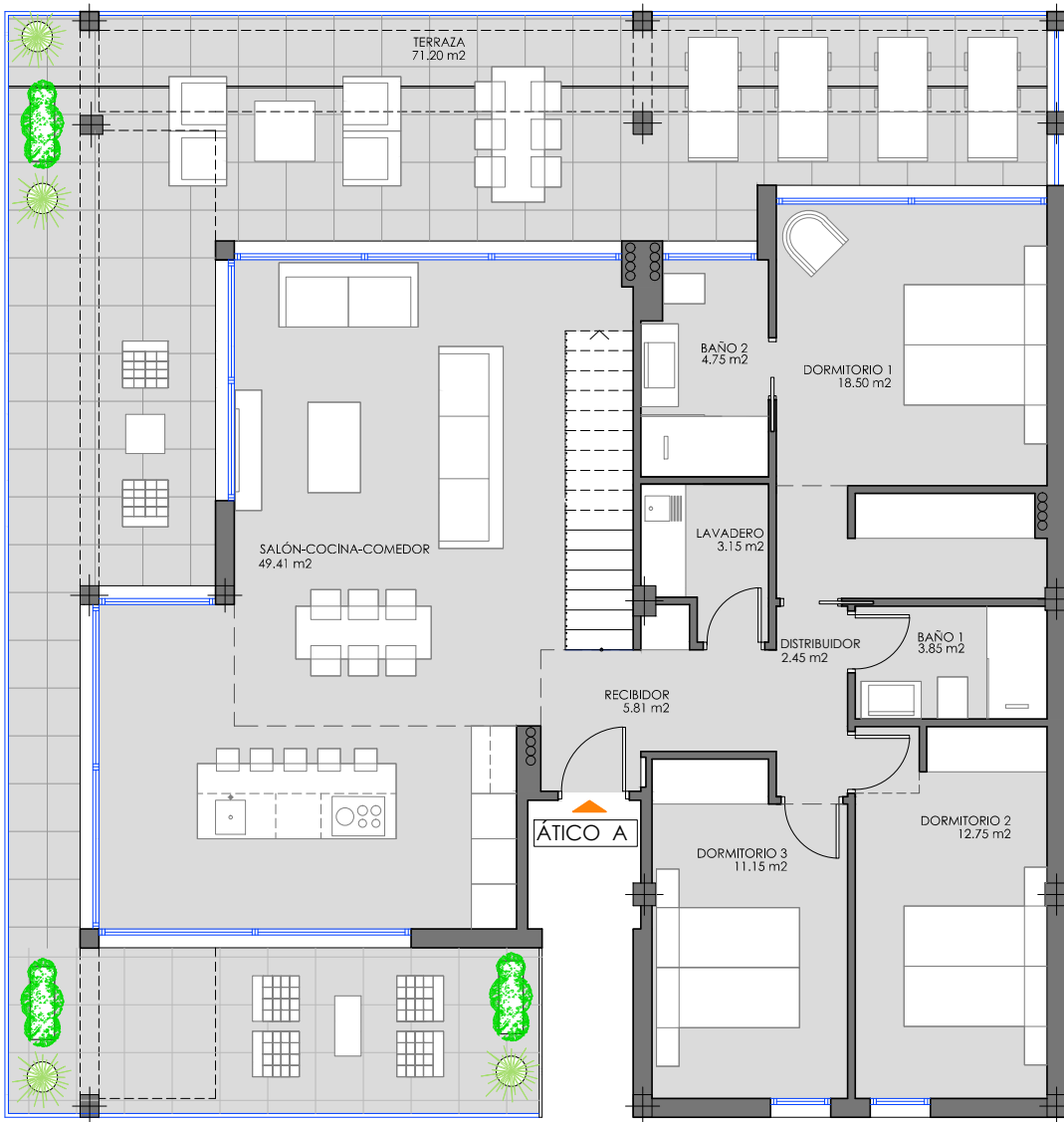
PLANTA ÁTICO
